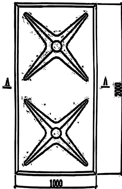
模块平面图
