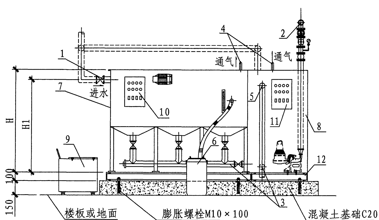
立面图
