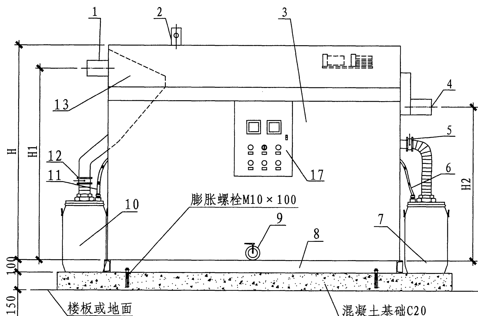
立面图
