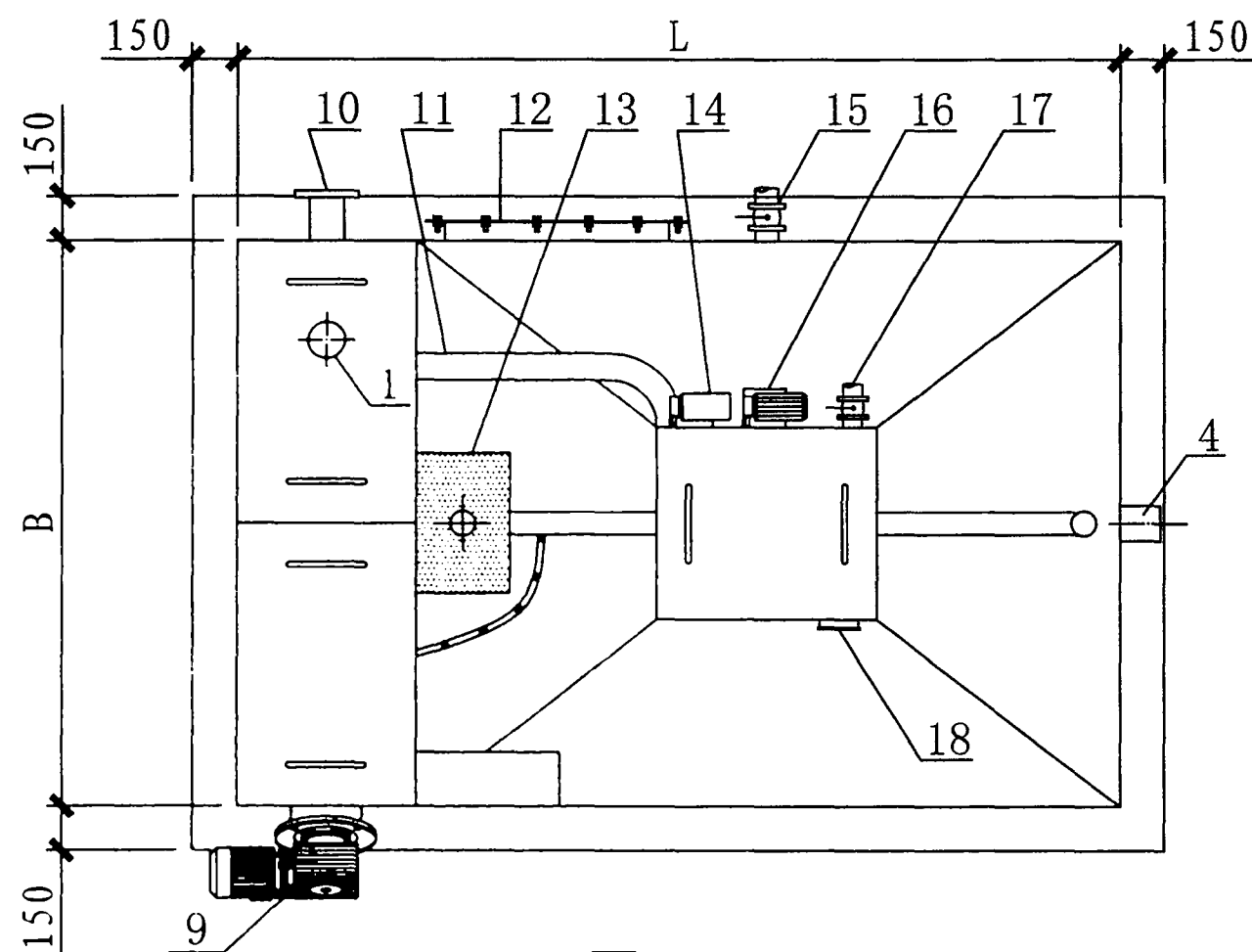
平面图
