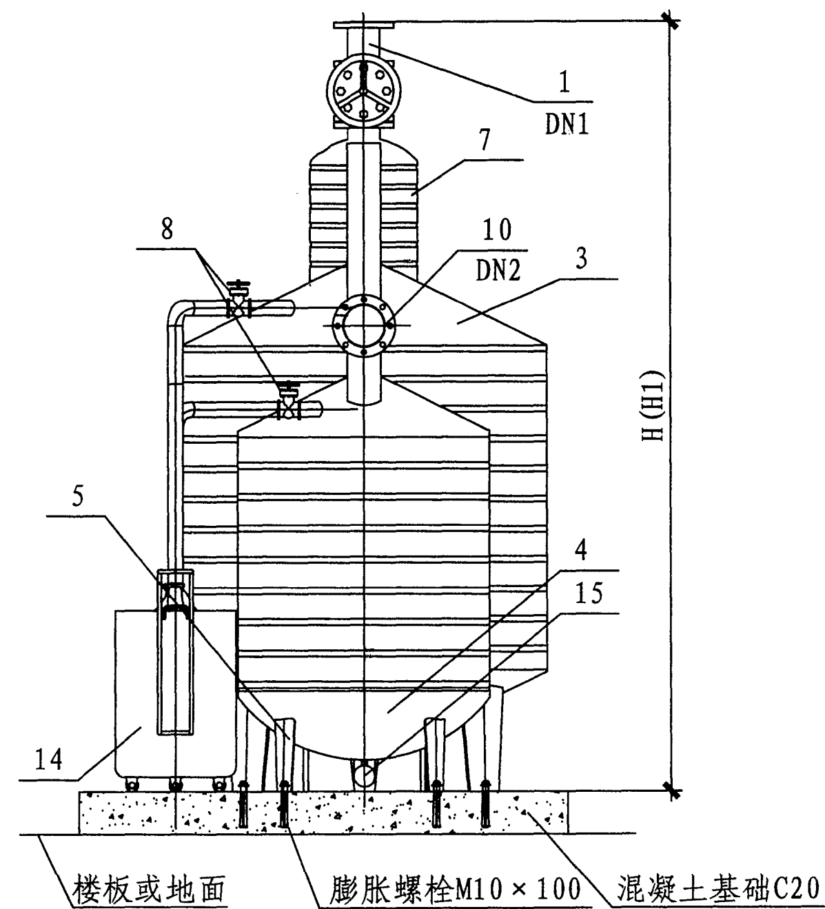
侧面图
