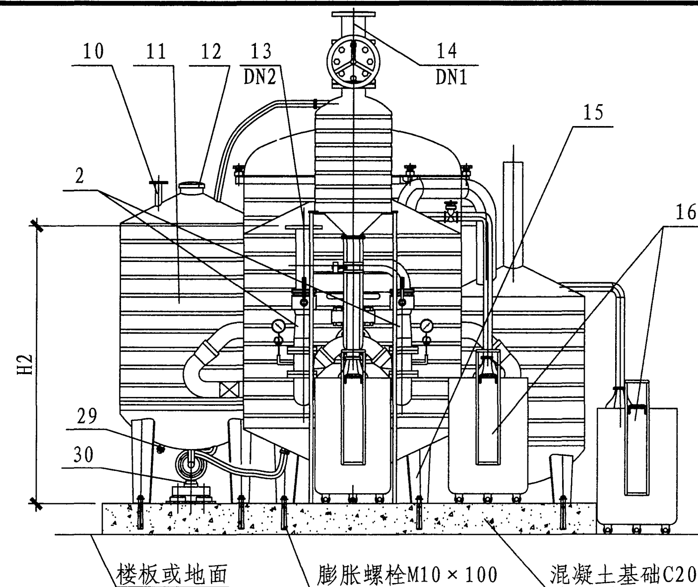
侧面图
