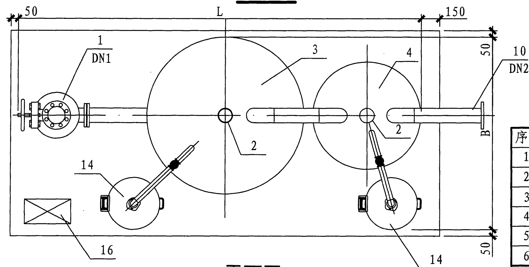
平面图
