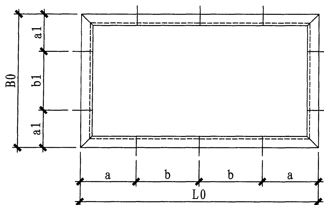
预埋件平面图
