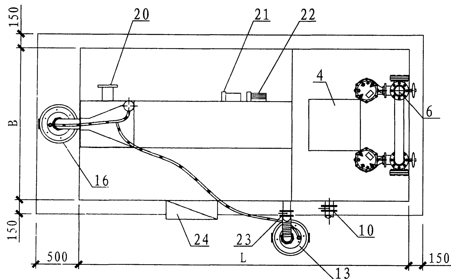
平面图
