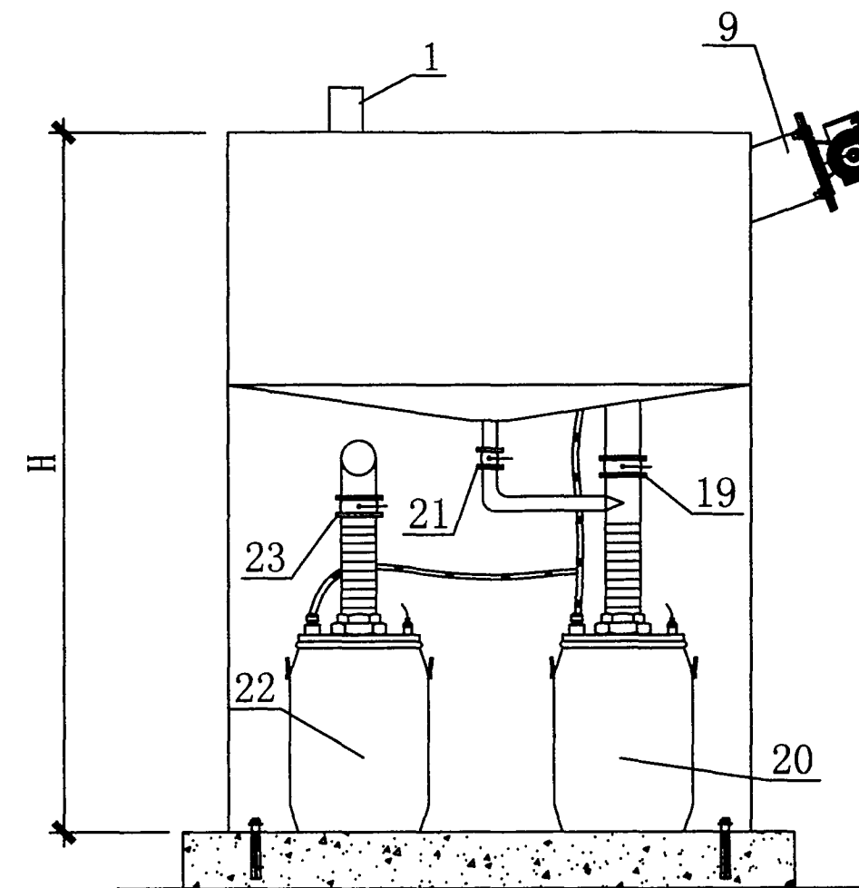
侧面图
