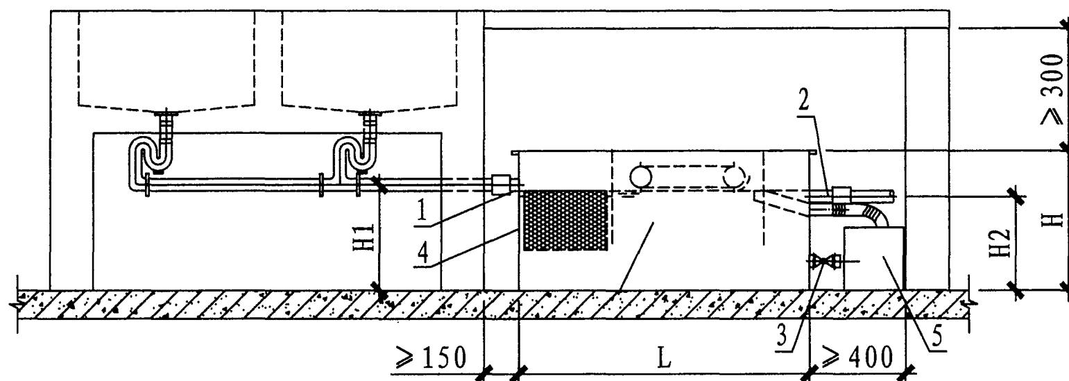
JYGYQ-D2安装立面图
