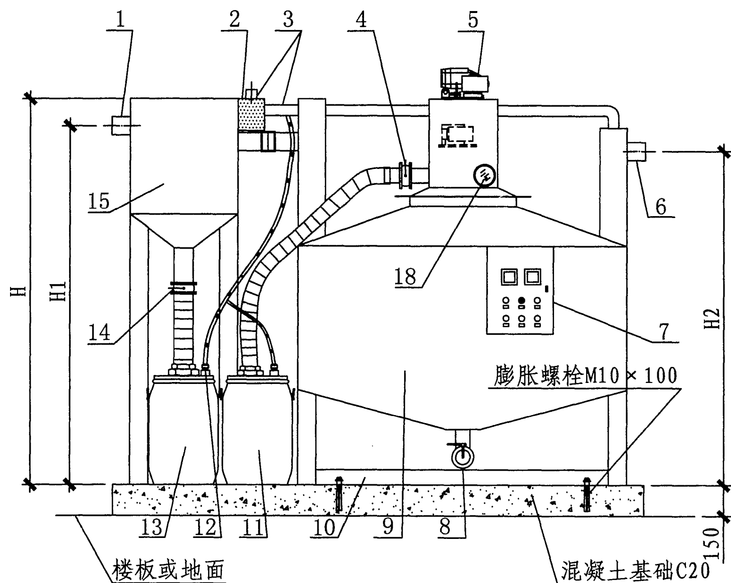
立面图
