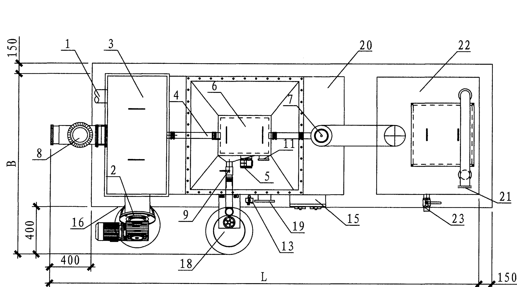
平面图
