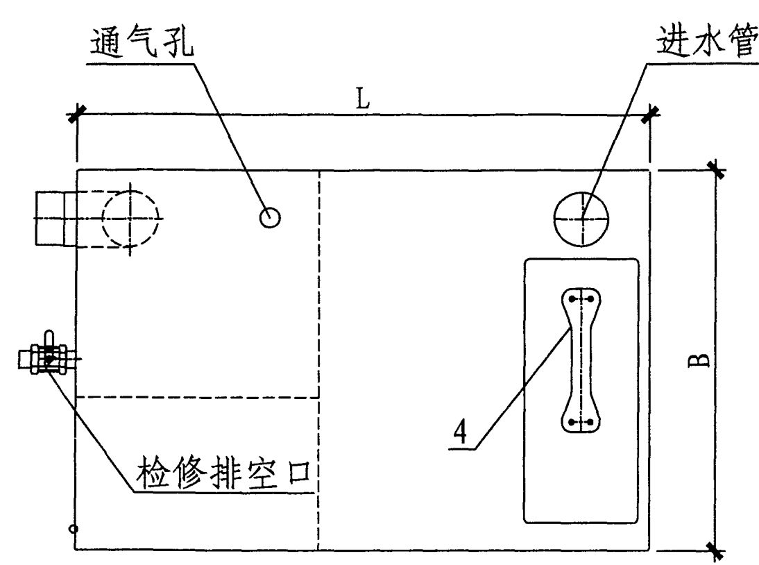
平面图
