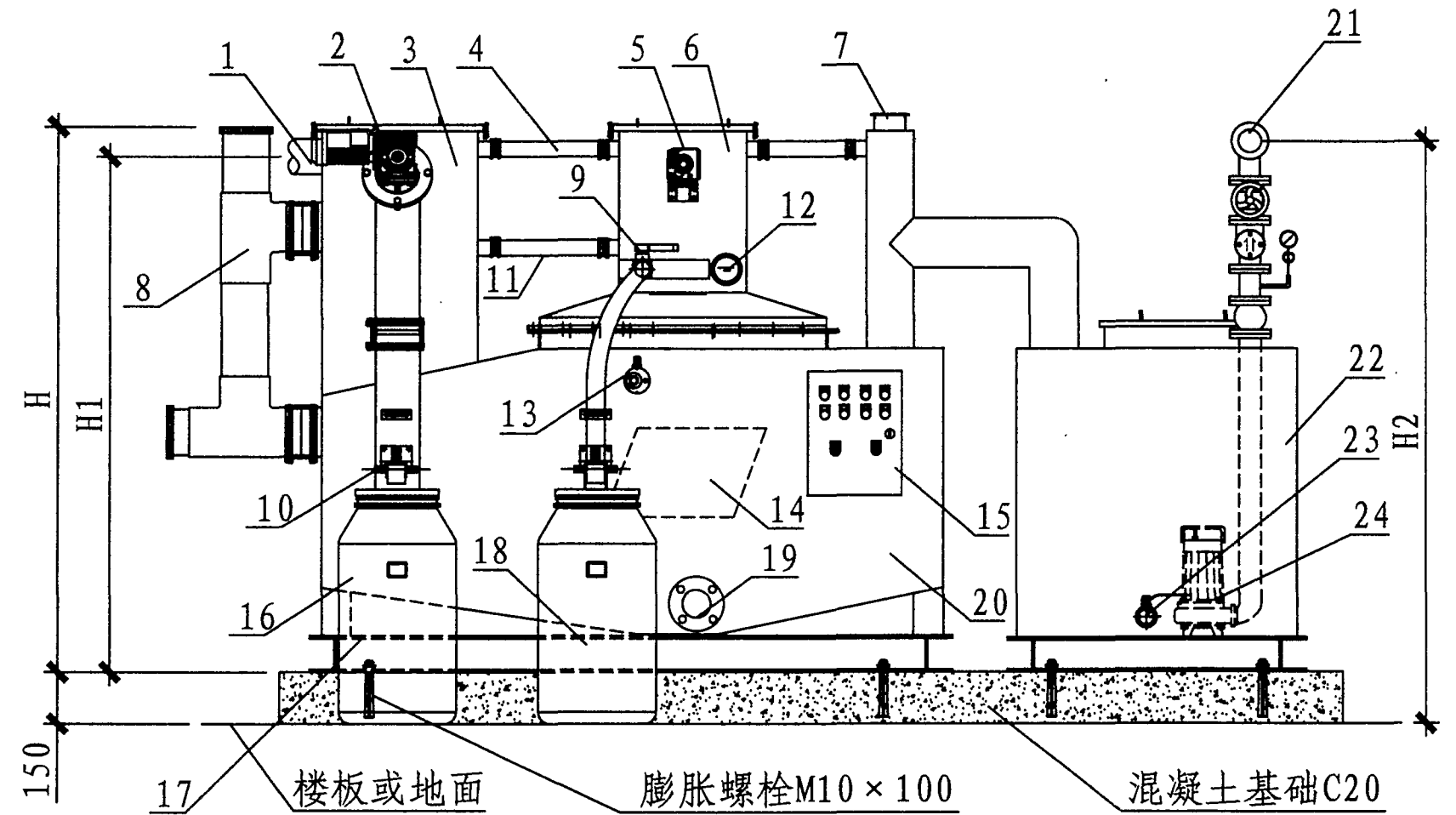
立面图
