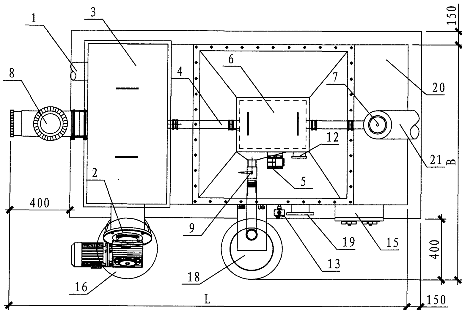
平面图
