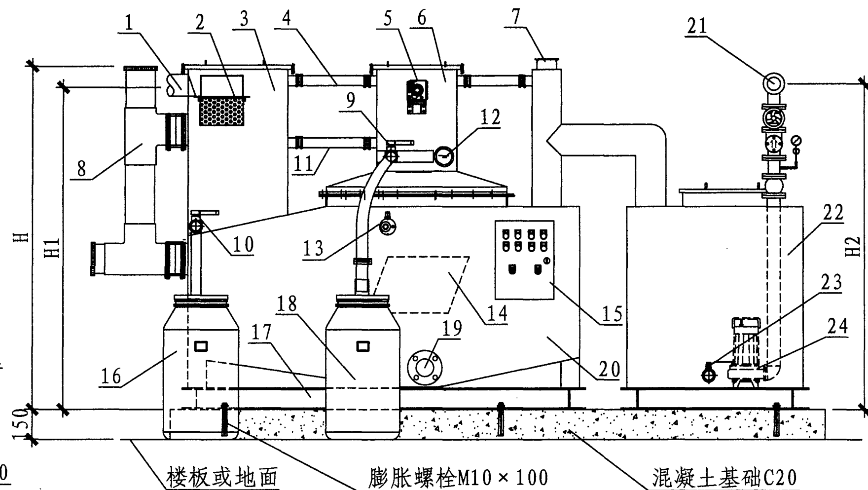
立面图
