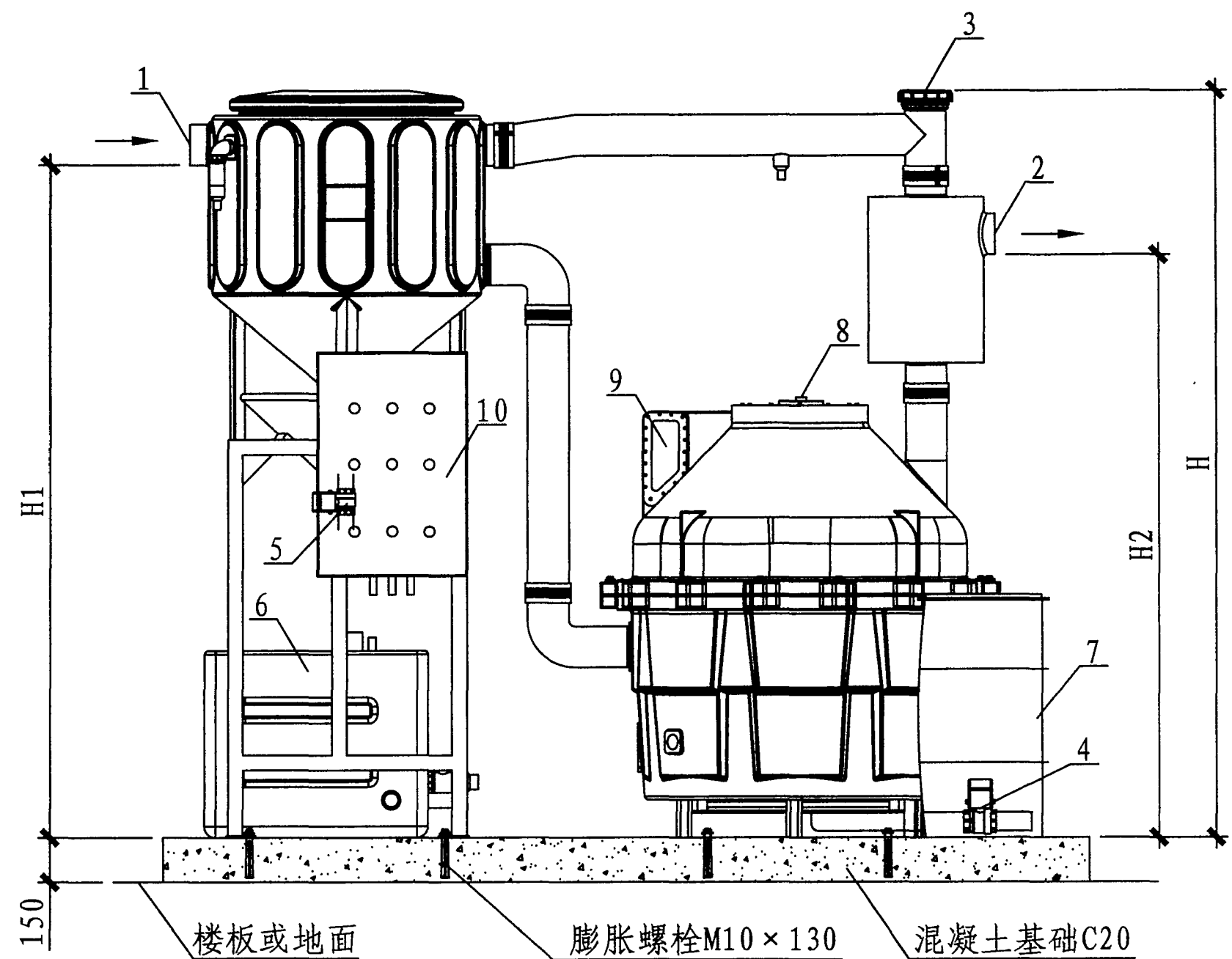
立面图
