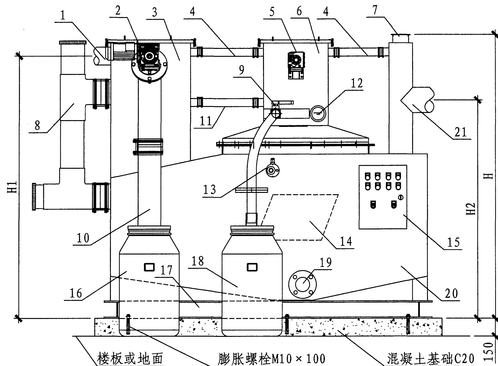
立面图
