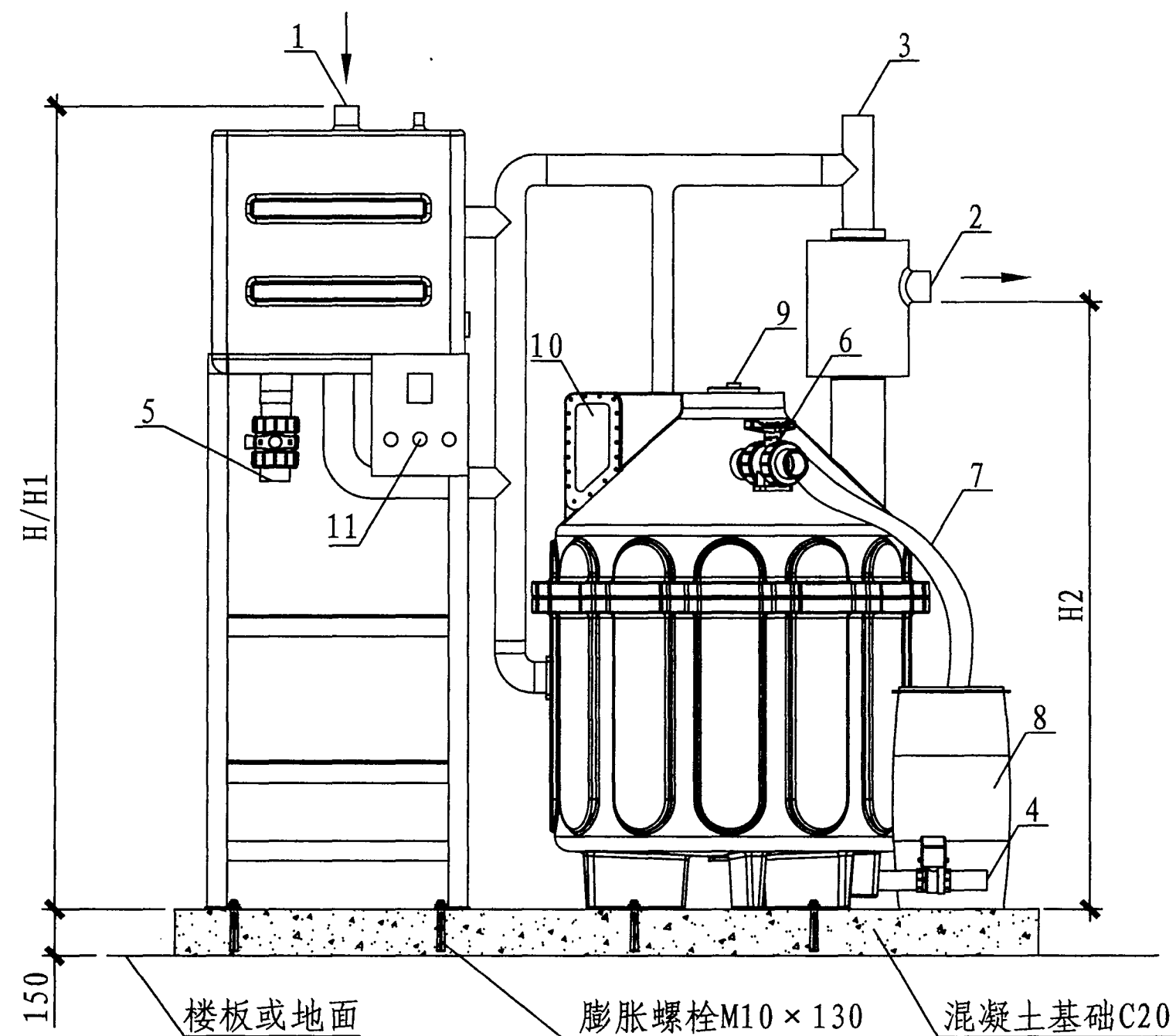
立面图
