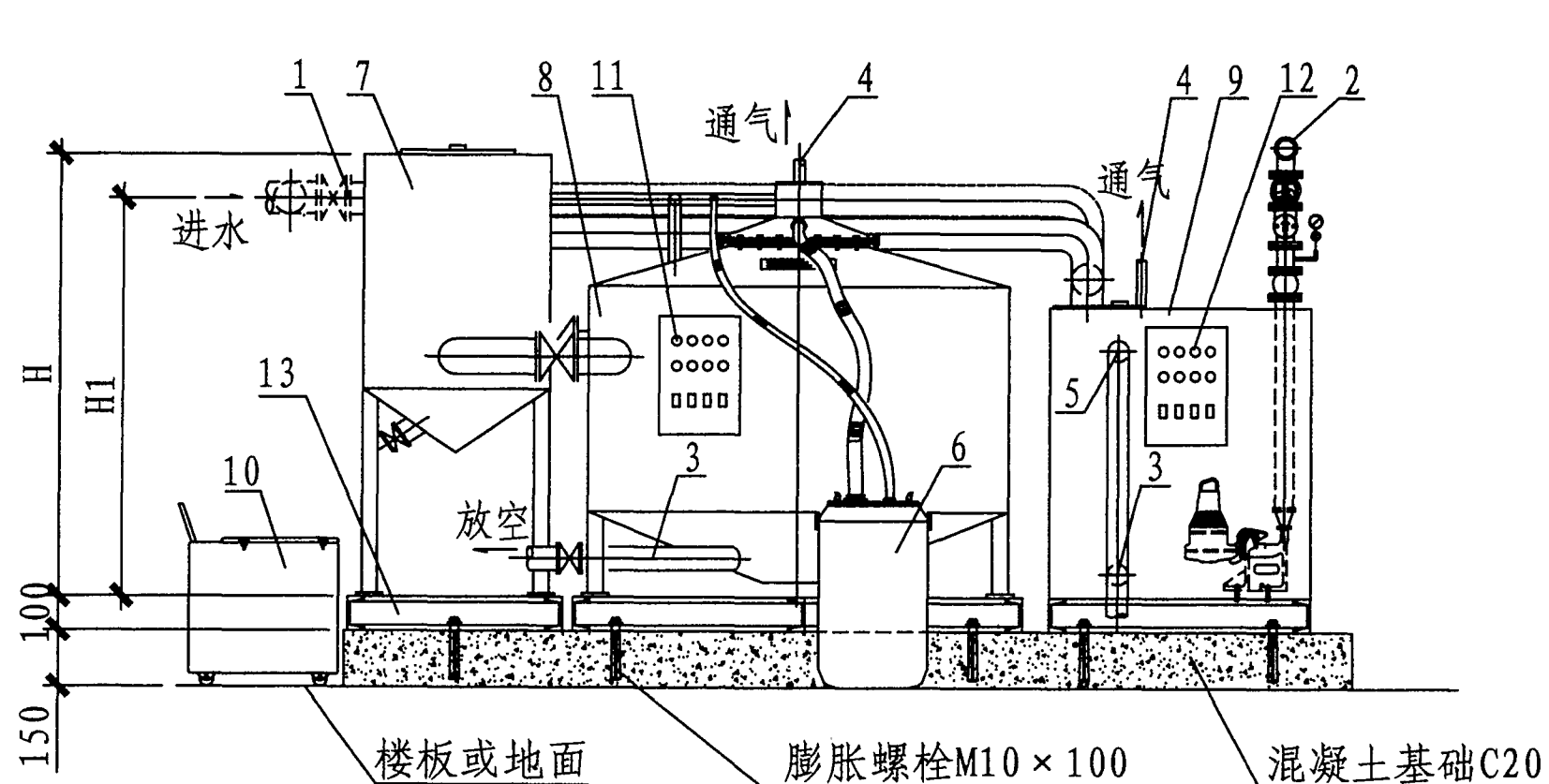
立面图
