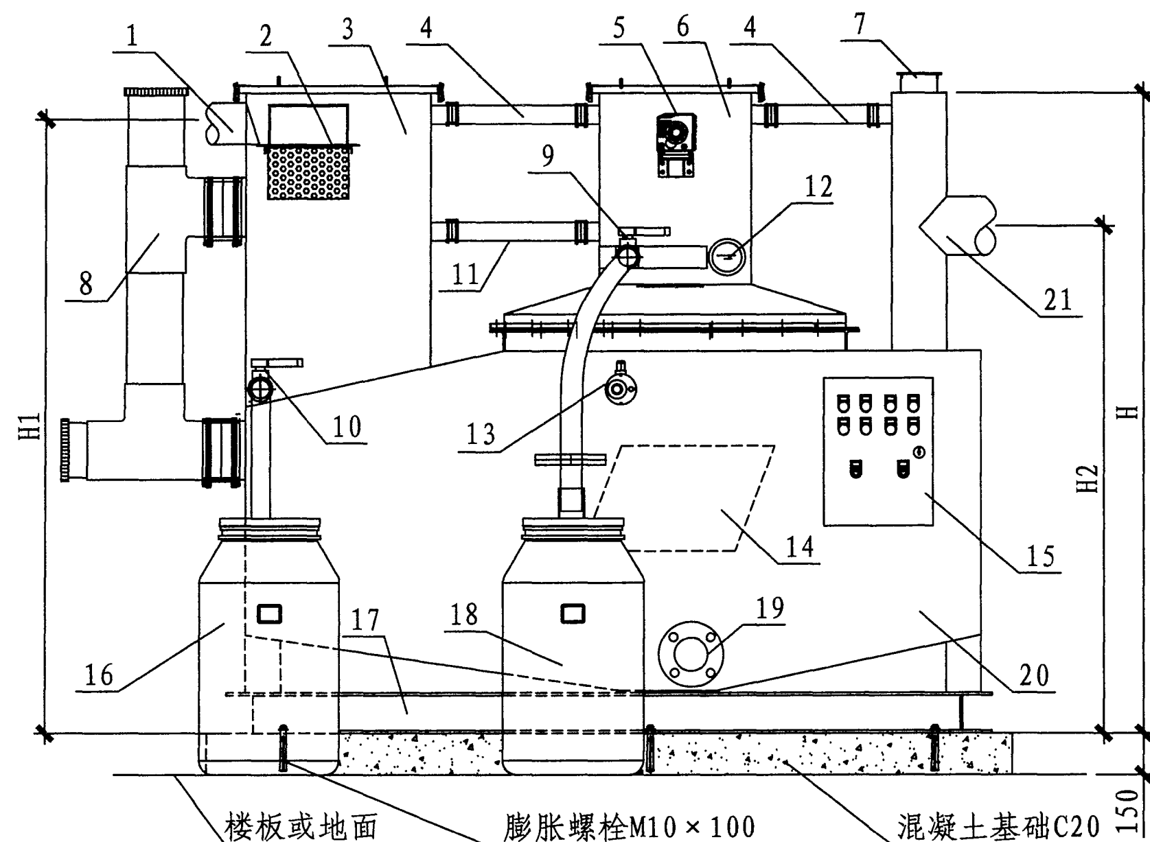
立面图
