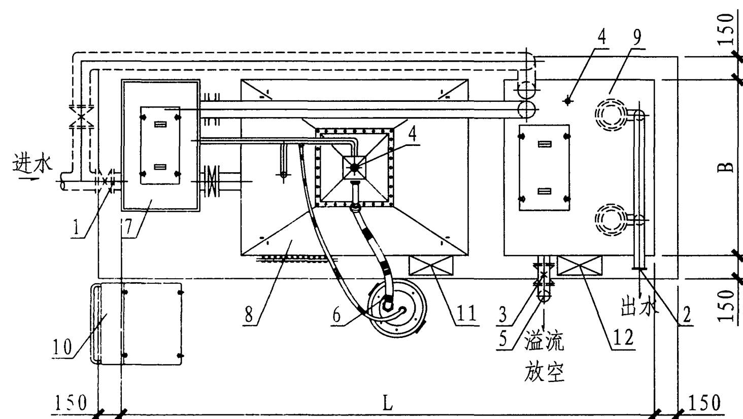
平面图
