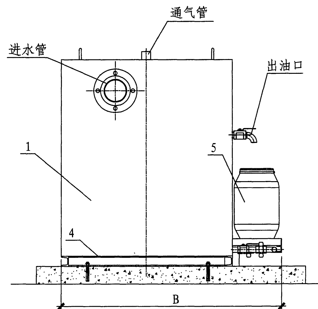
侧面图
