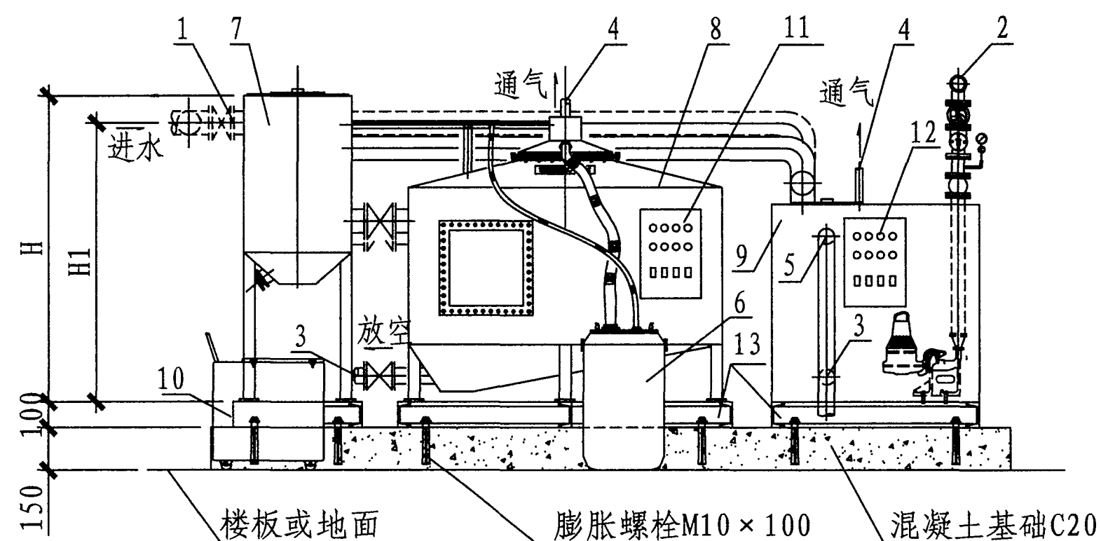
立面图
