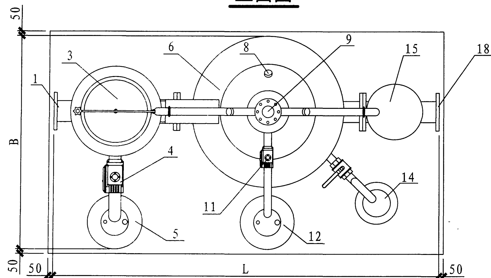
平面图
