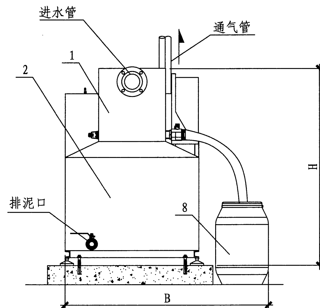
侧面图
