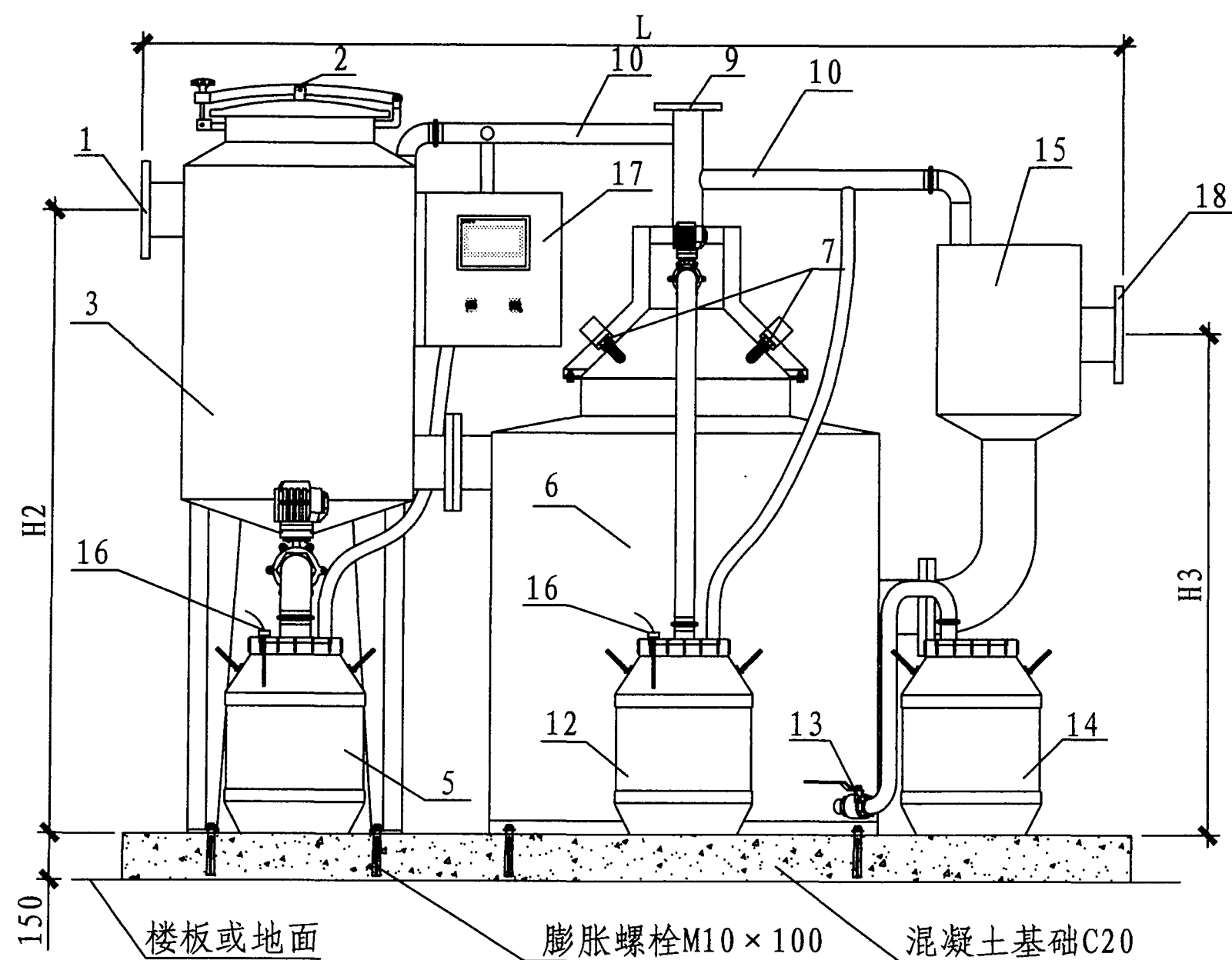
立面图
