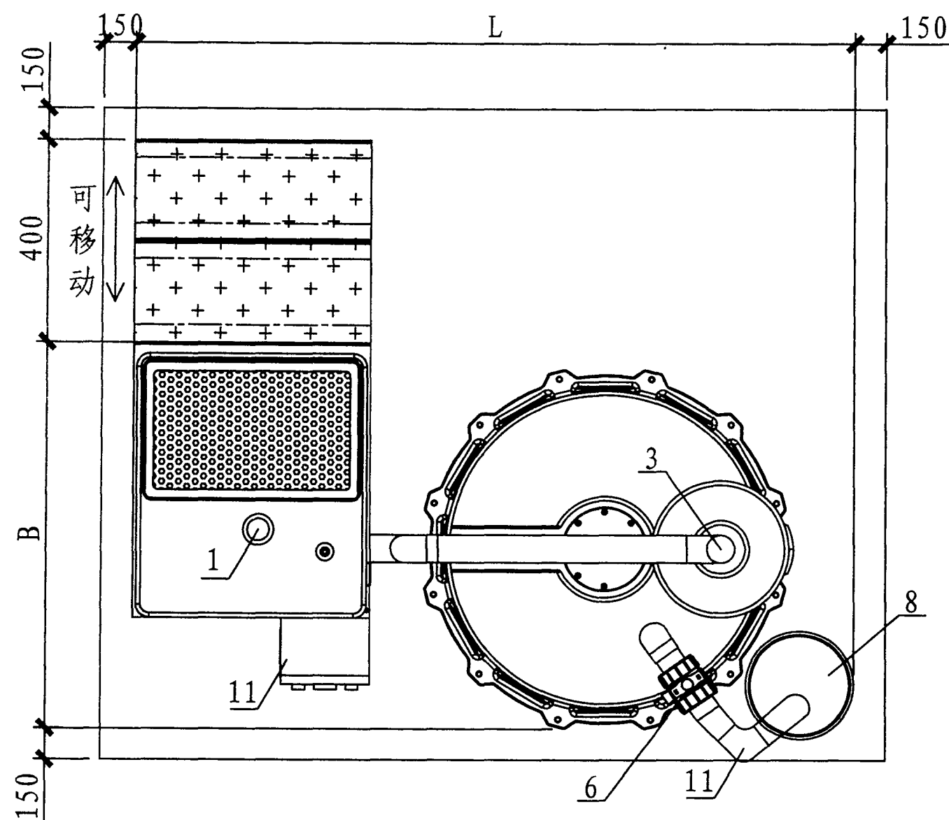
平面图
