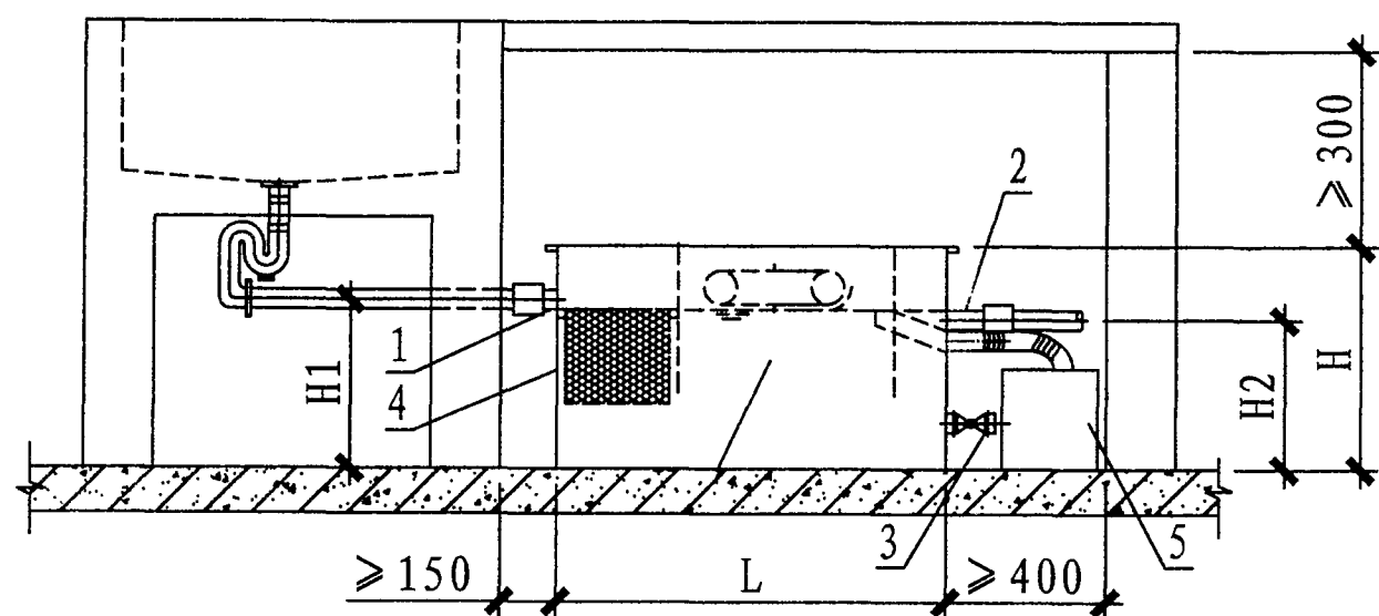
JYGYQ-D1安装立面图
