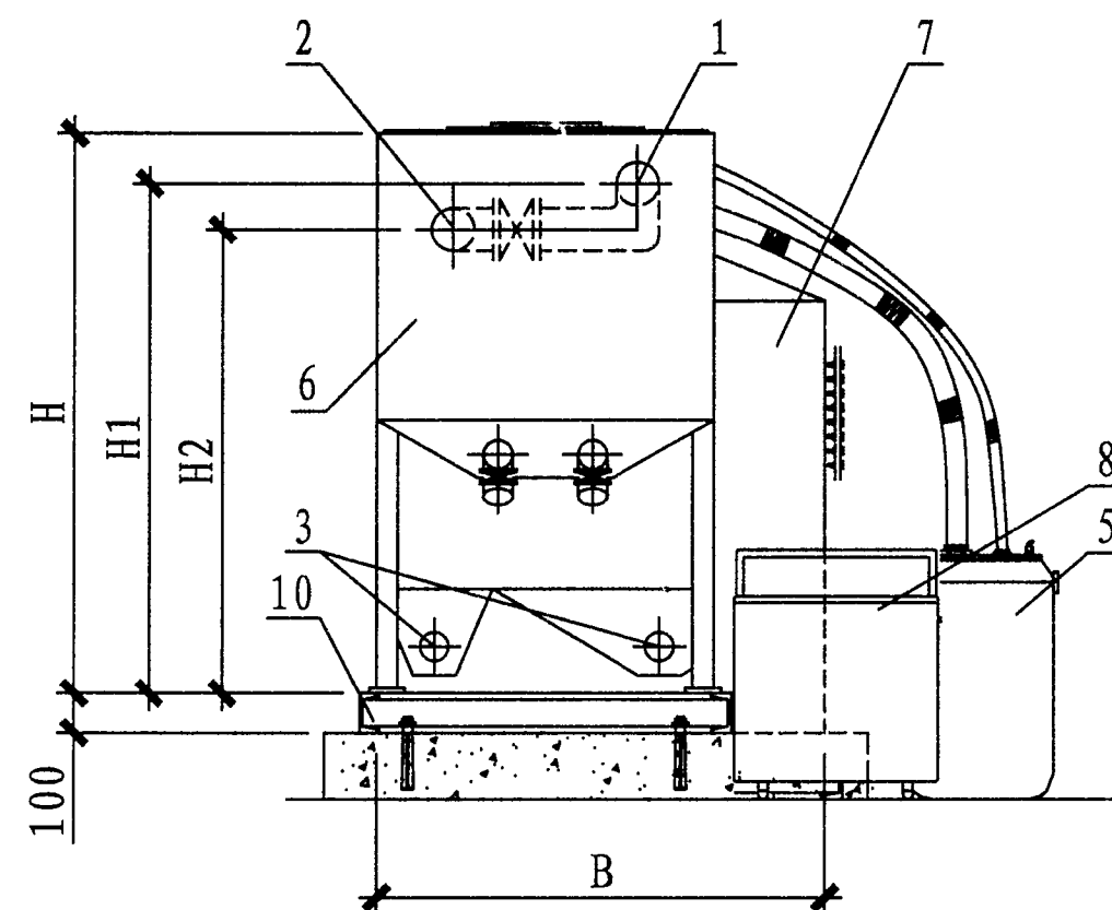
侧面图
