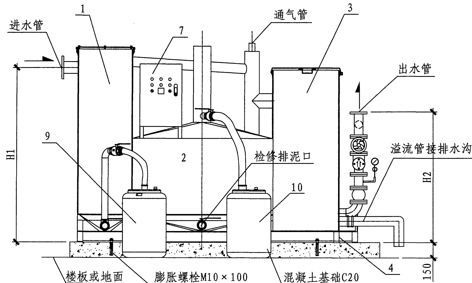
立面图
