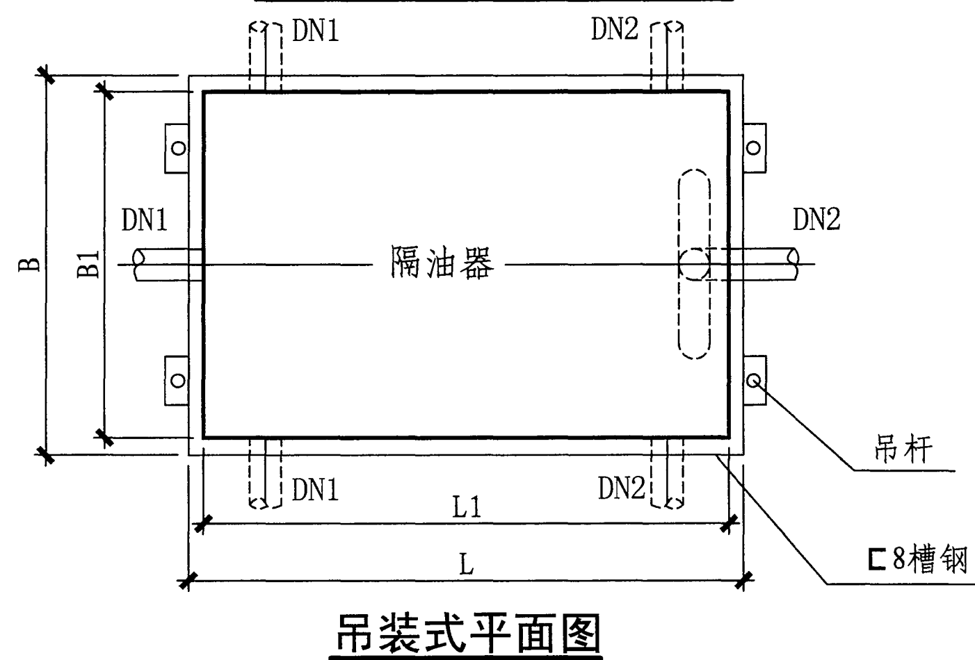
吊装式隔油器安装示意图
