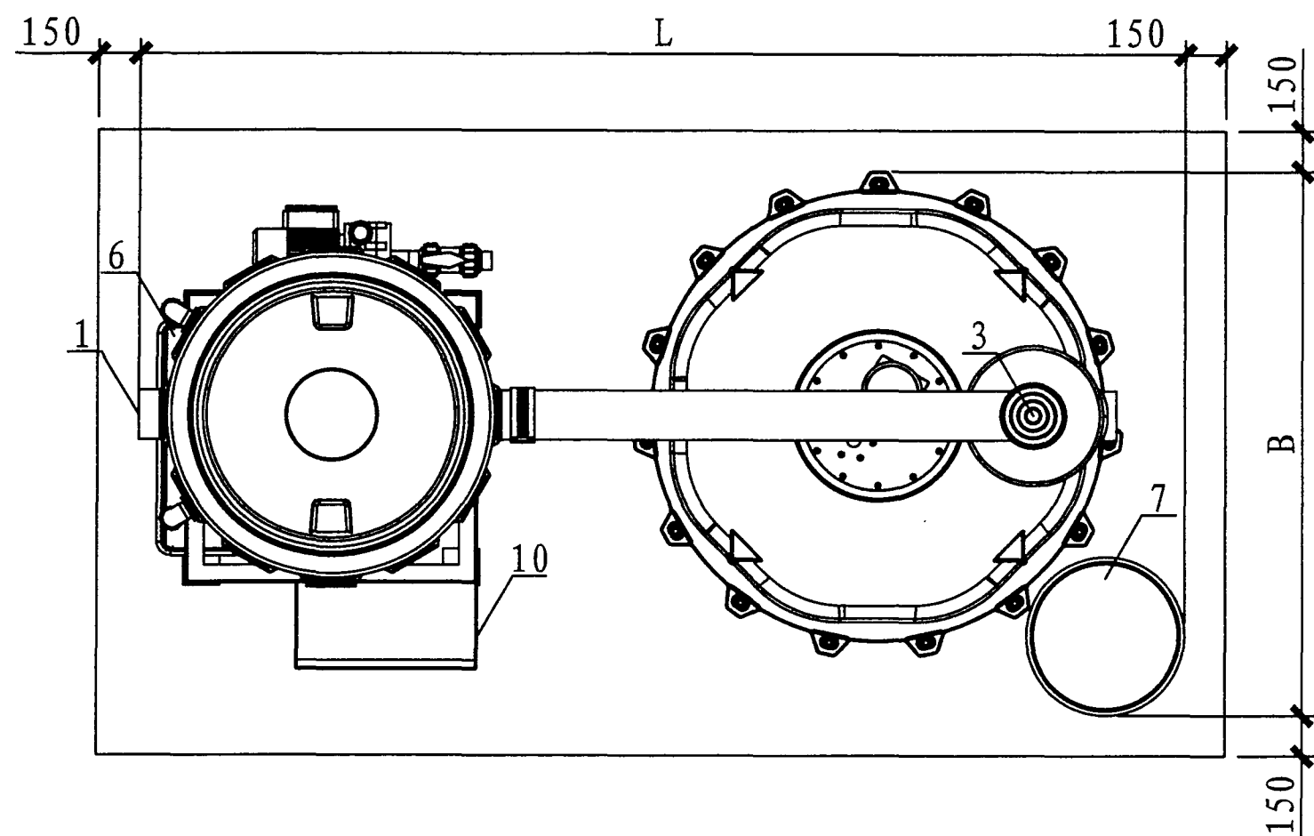
平面图
