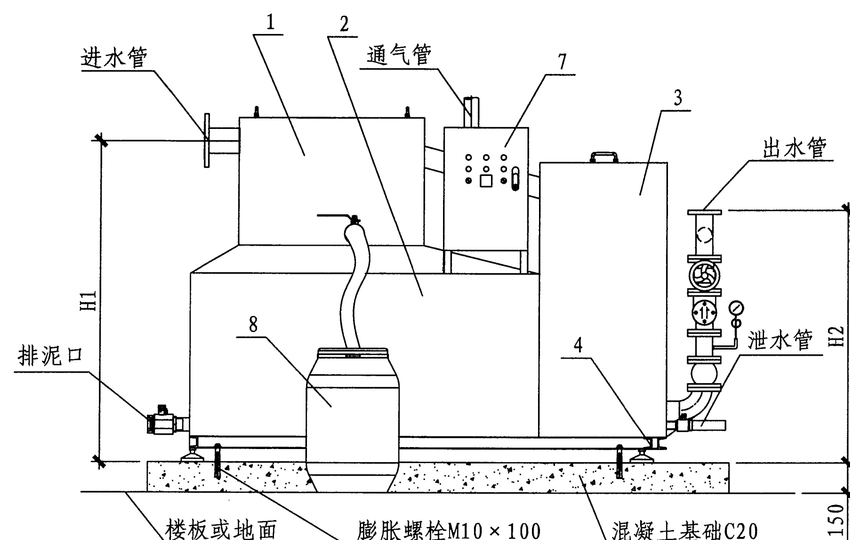
立面图
