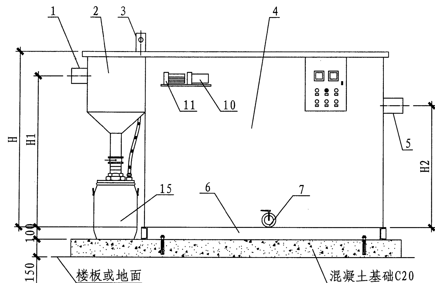
立面图
