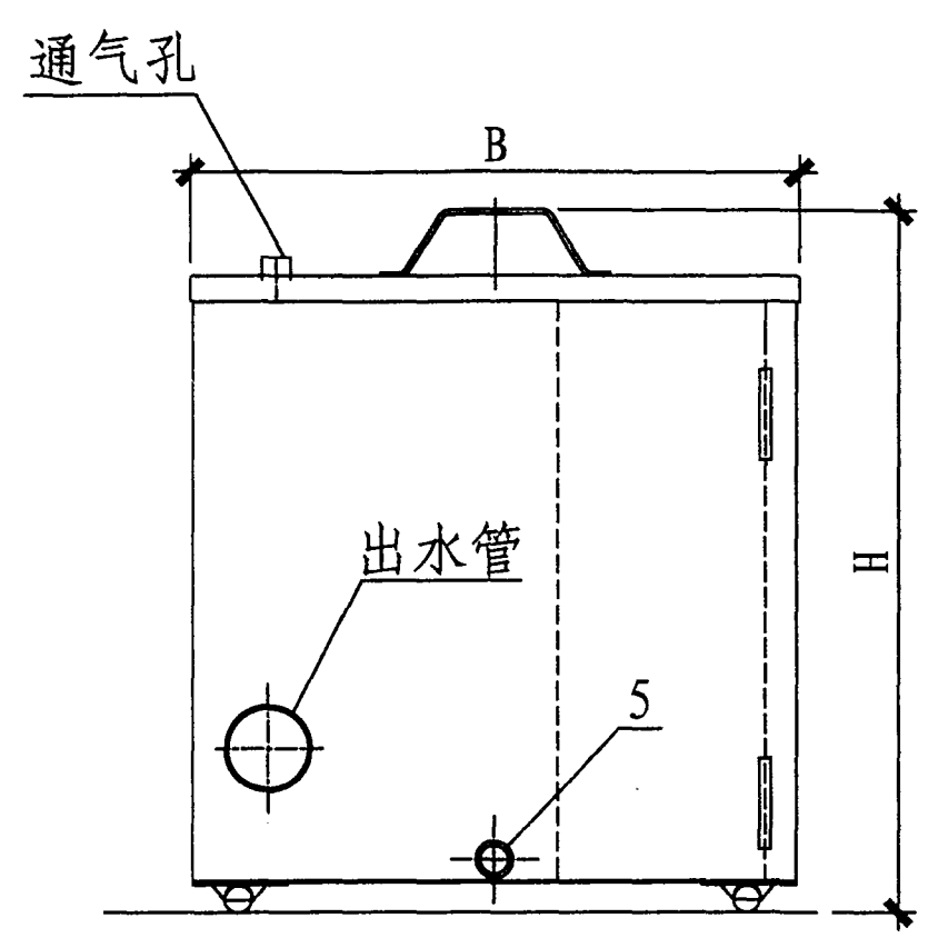
侧面图
