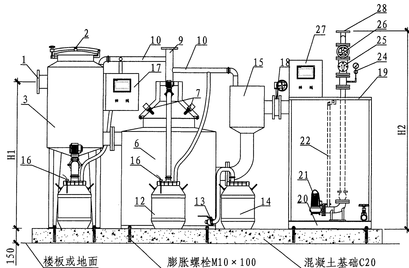
立面图
