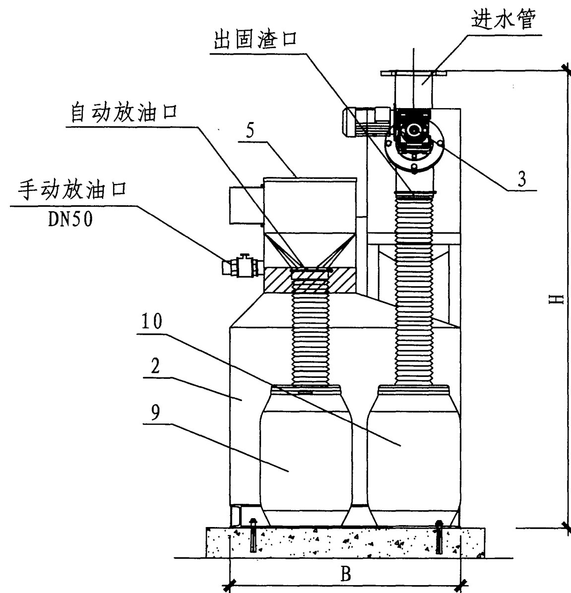
侧面图
