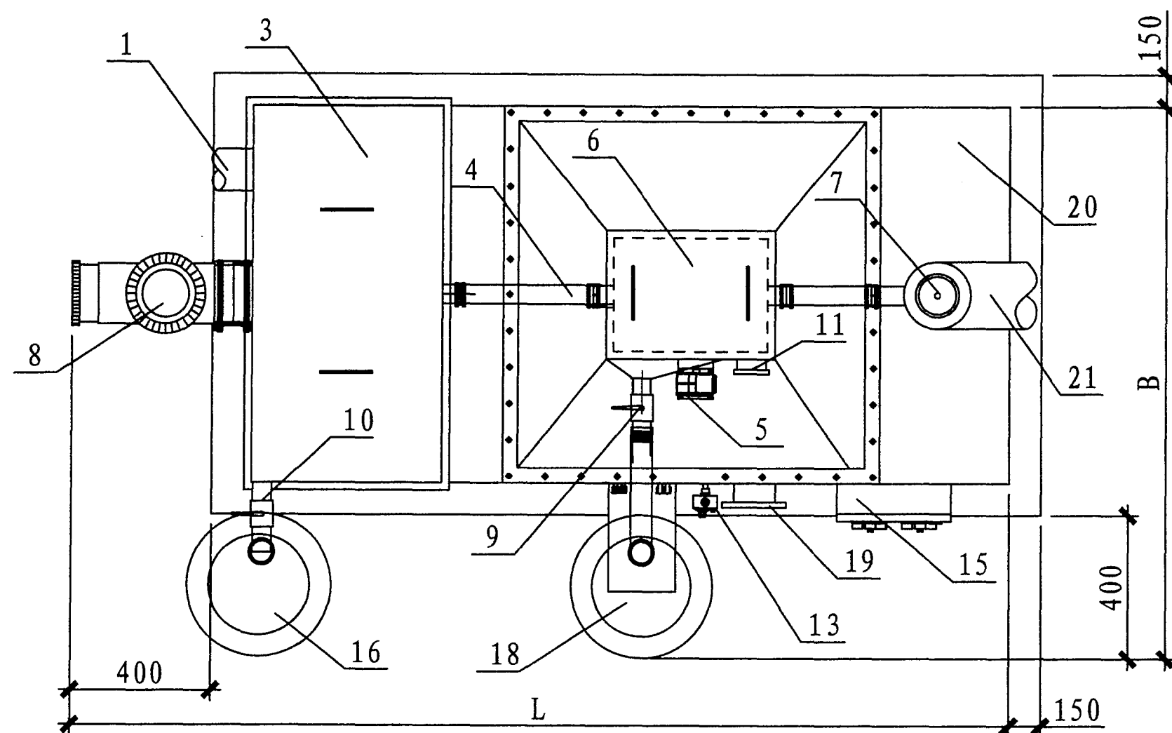
平面图
