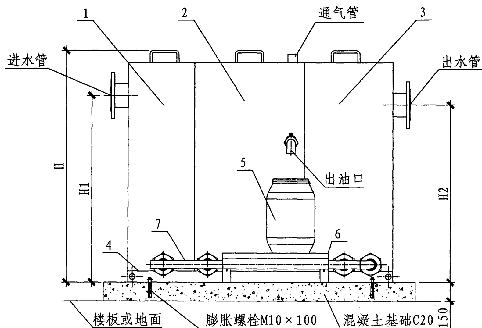
立面图
