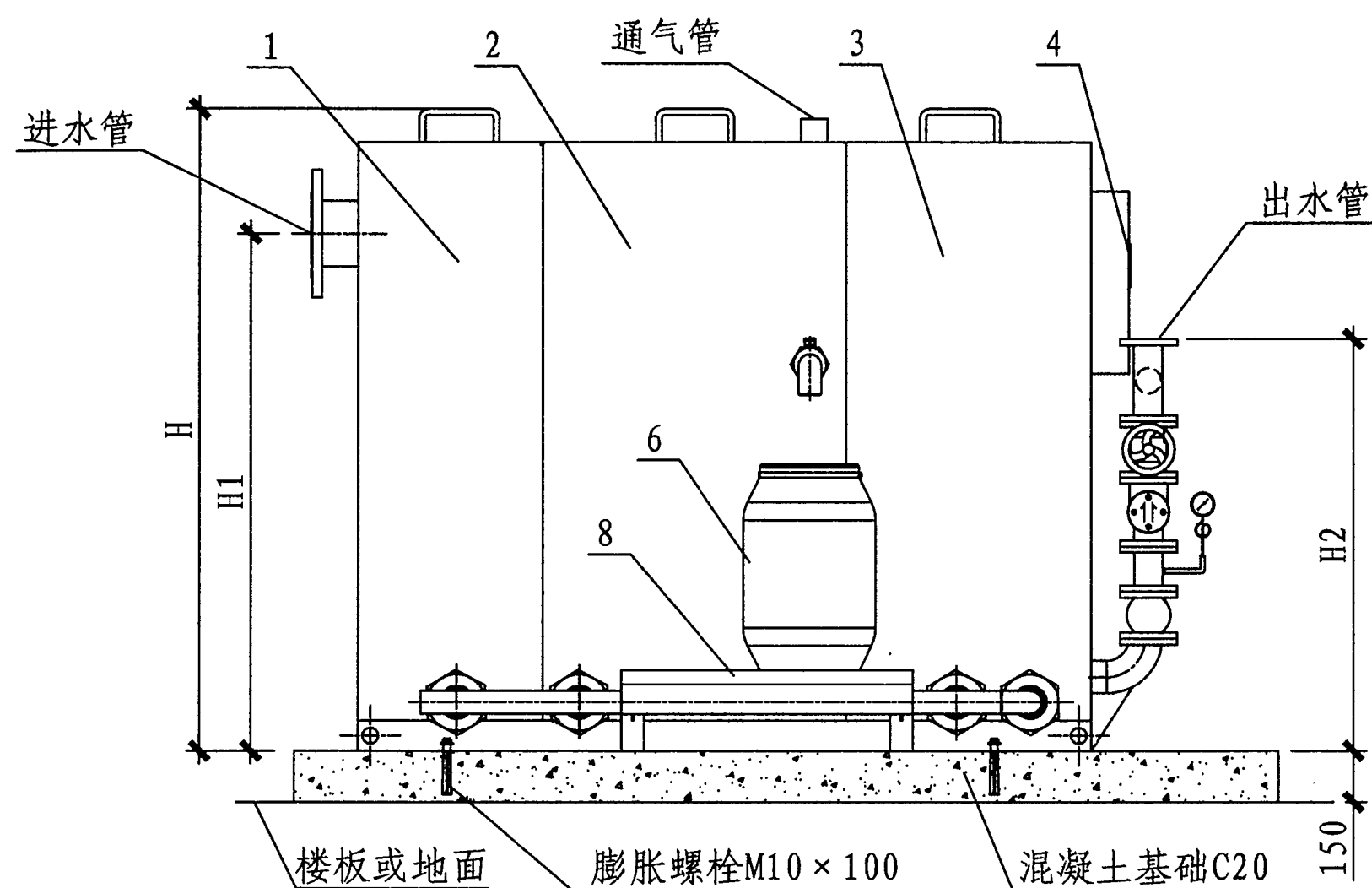
立面图
