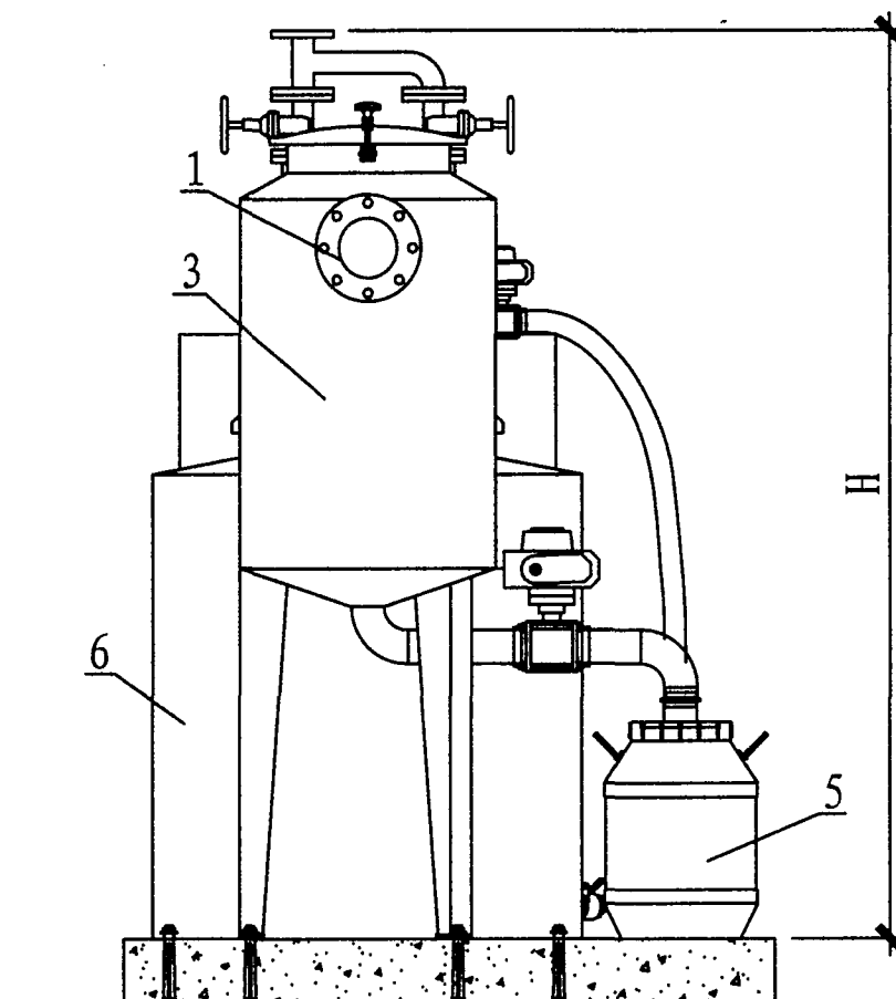
侧面图
