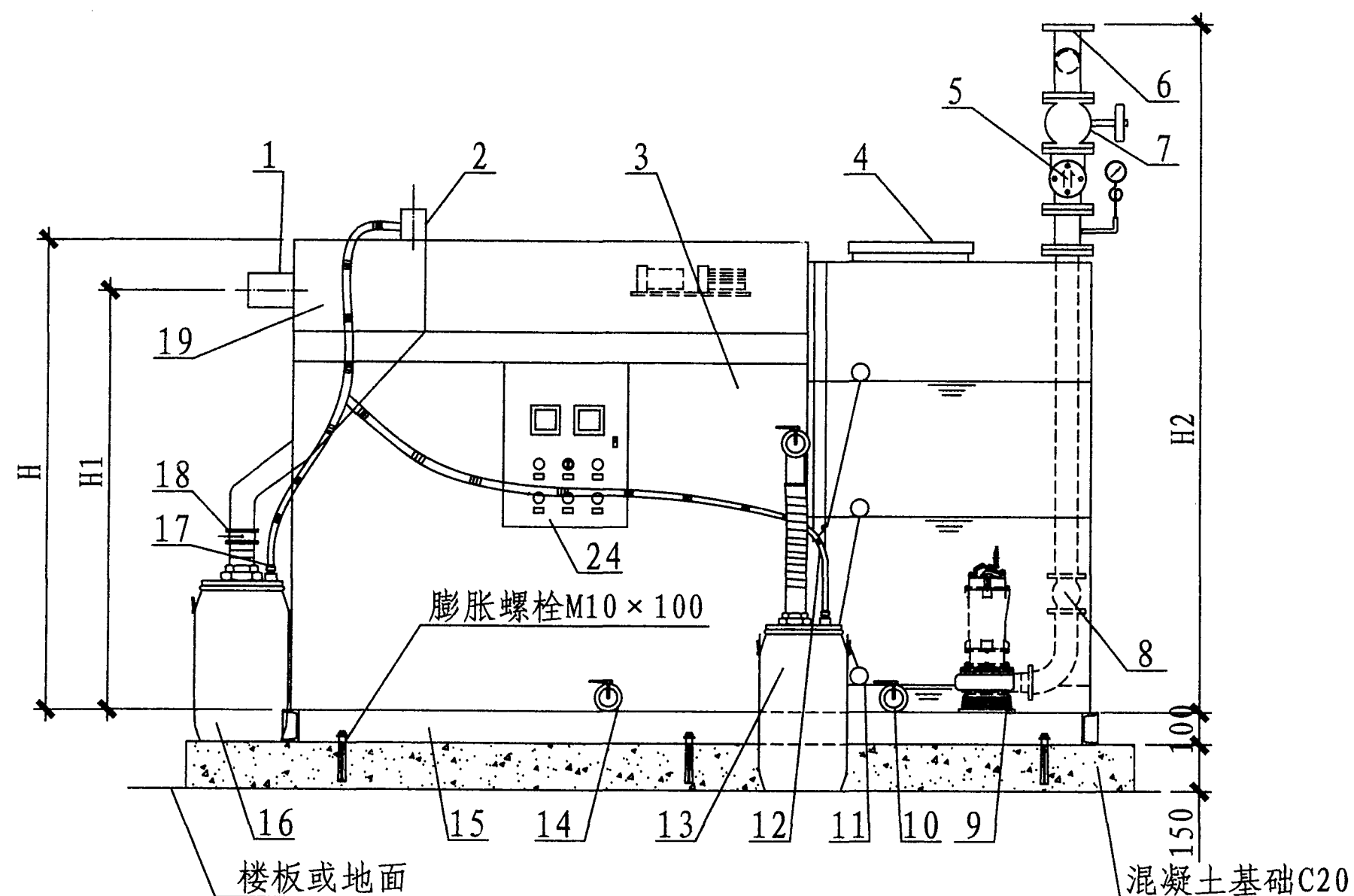
立面图
