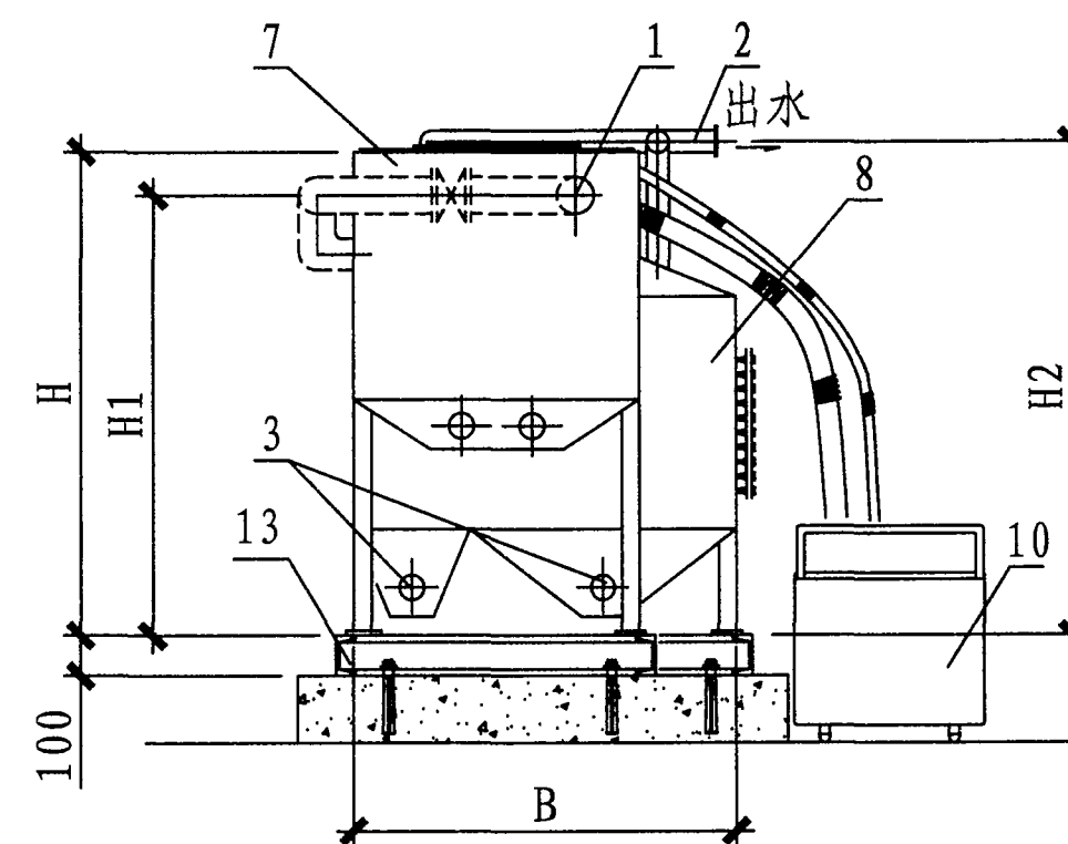
侧面图
