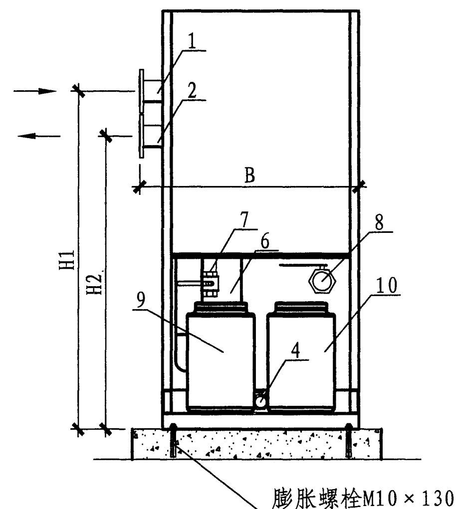
左视图
