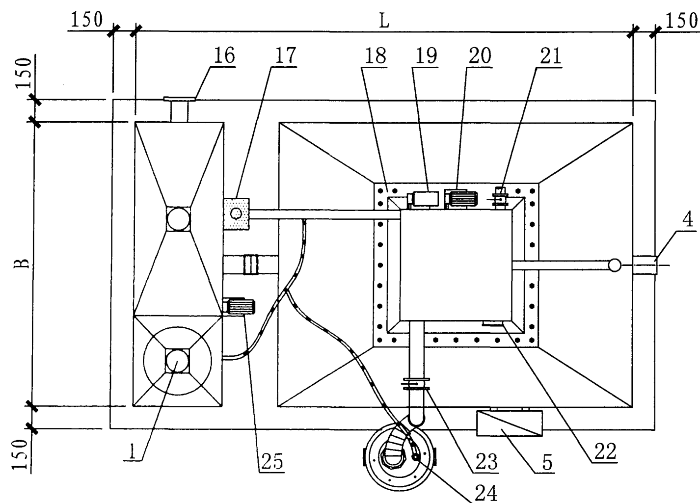
平面图
