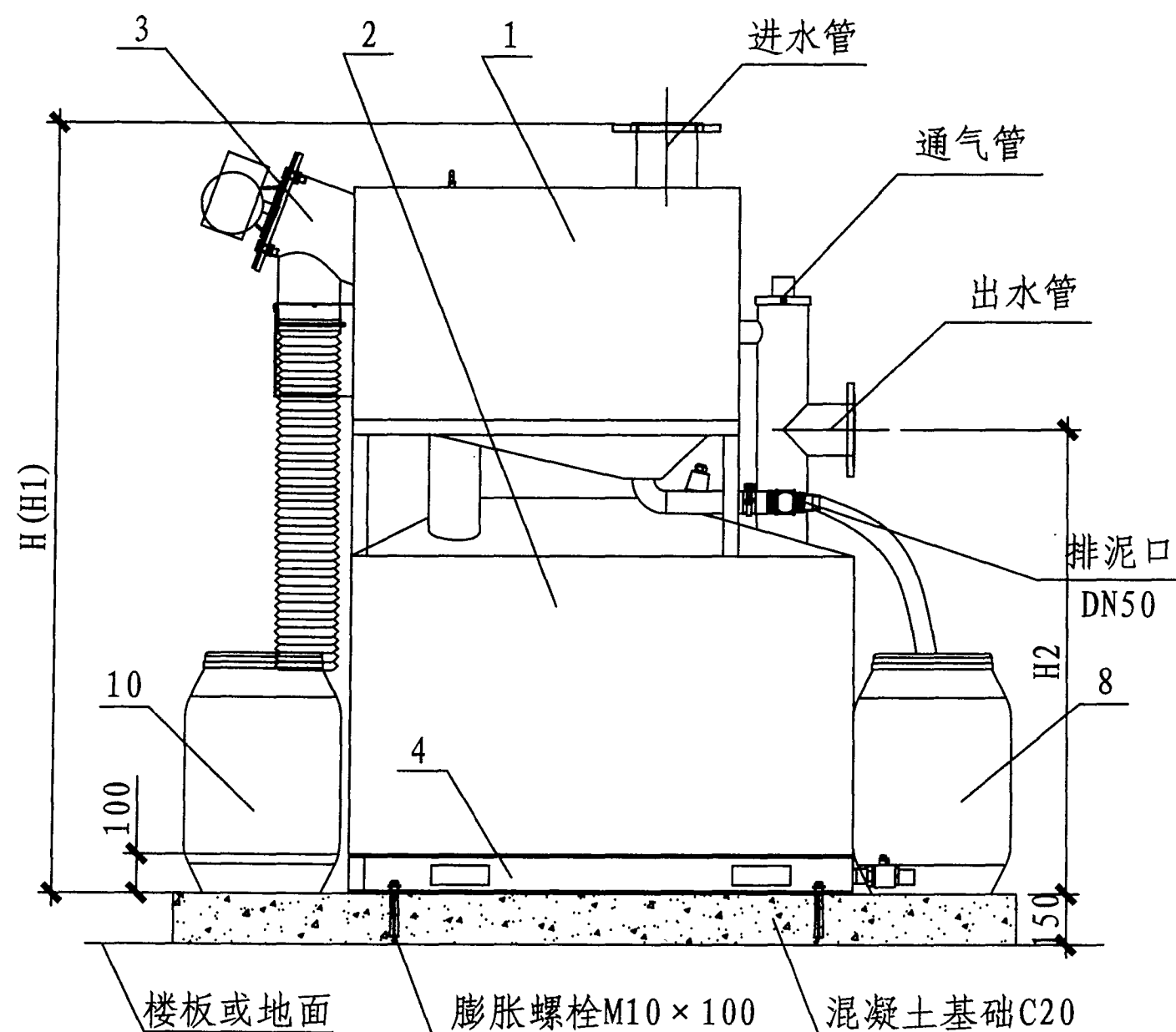
立面图
