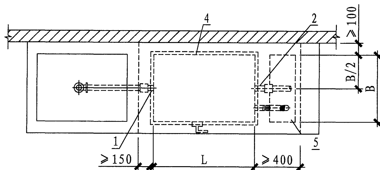
JYGYQ-D1安装平面图
