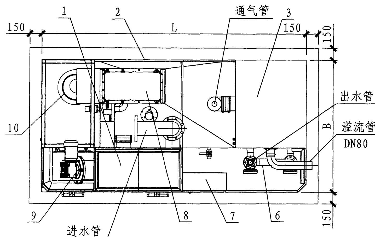
平面图
