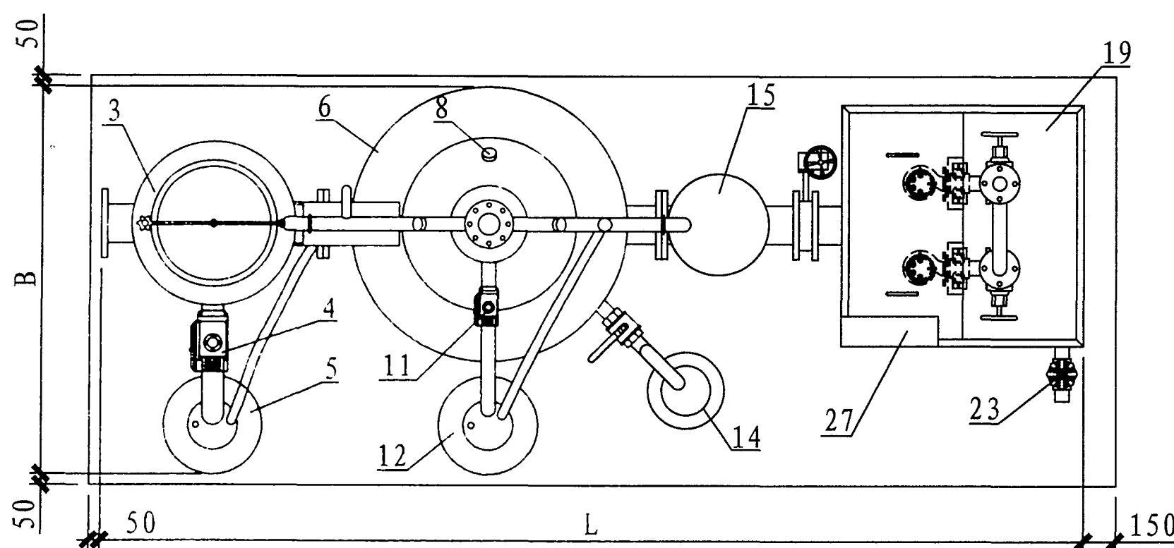
平面图
