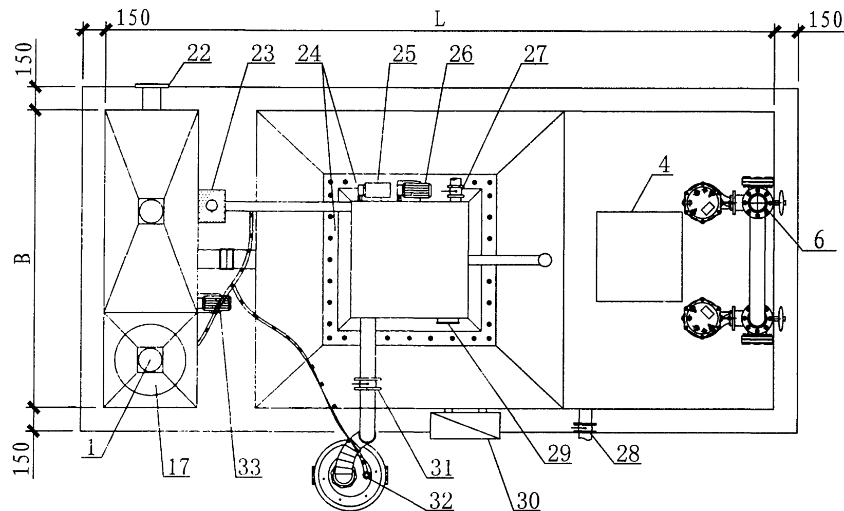
平面图
