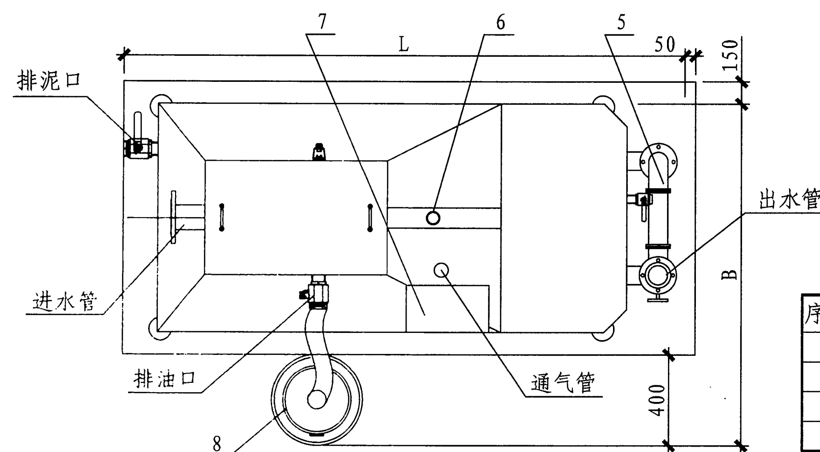
平面图
