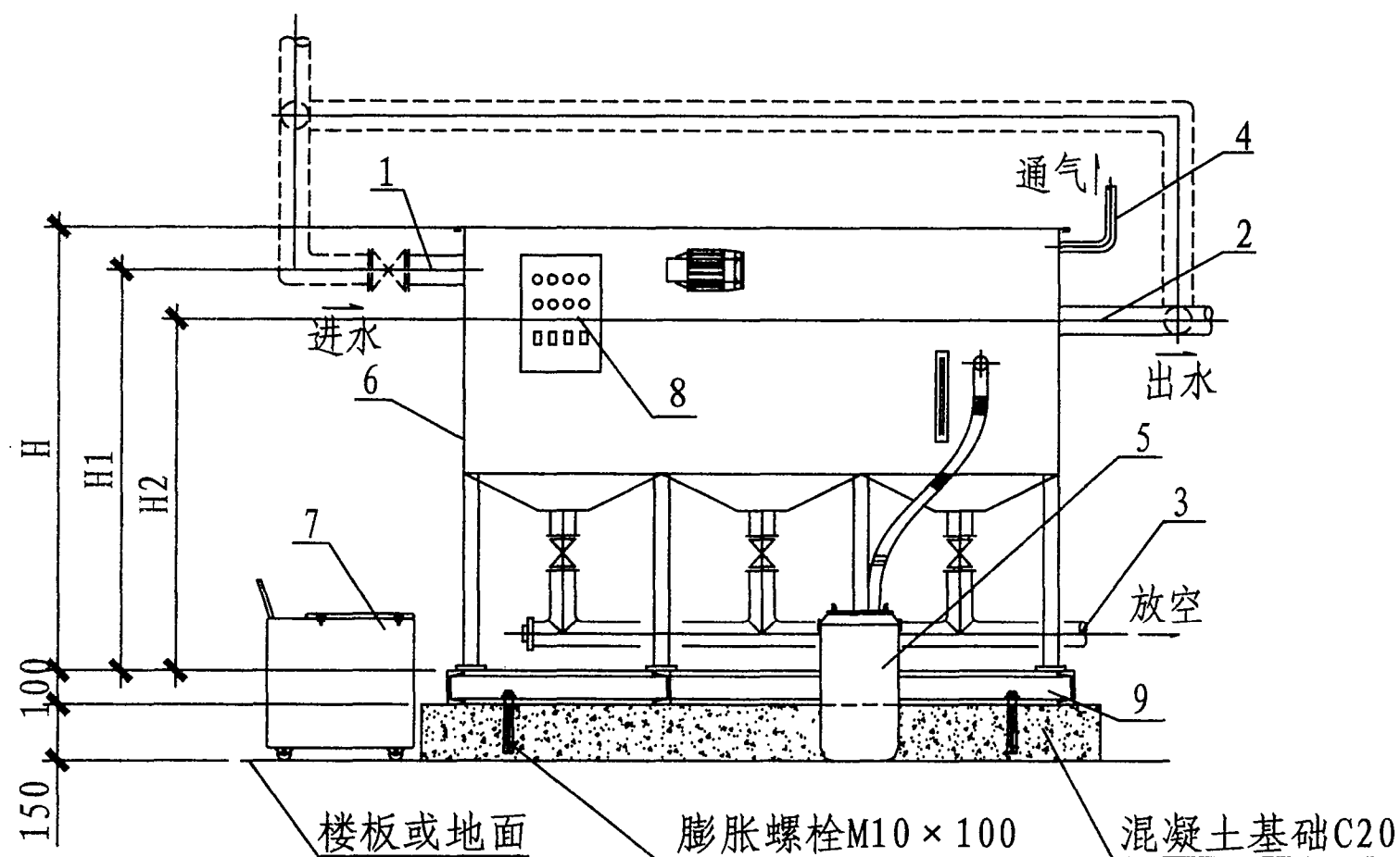
立面图
