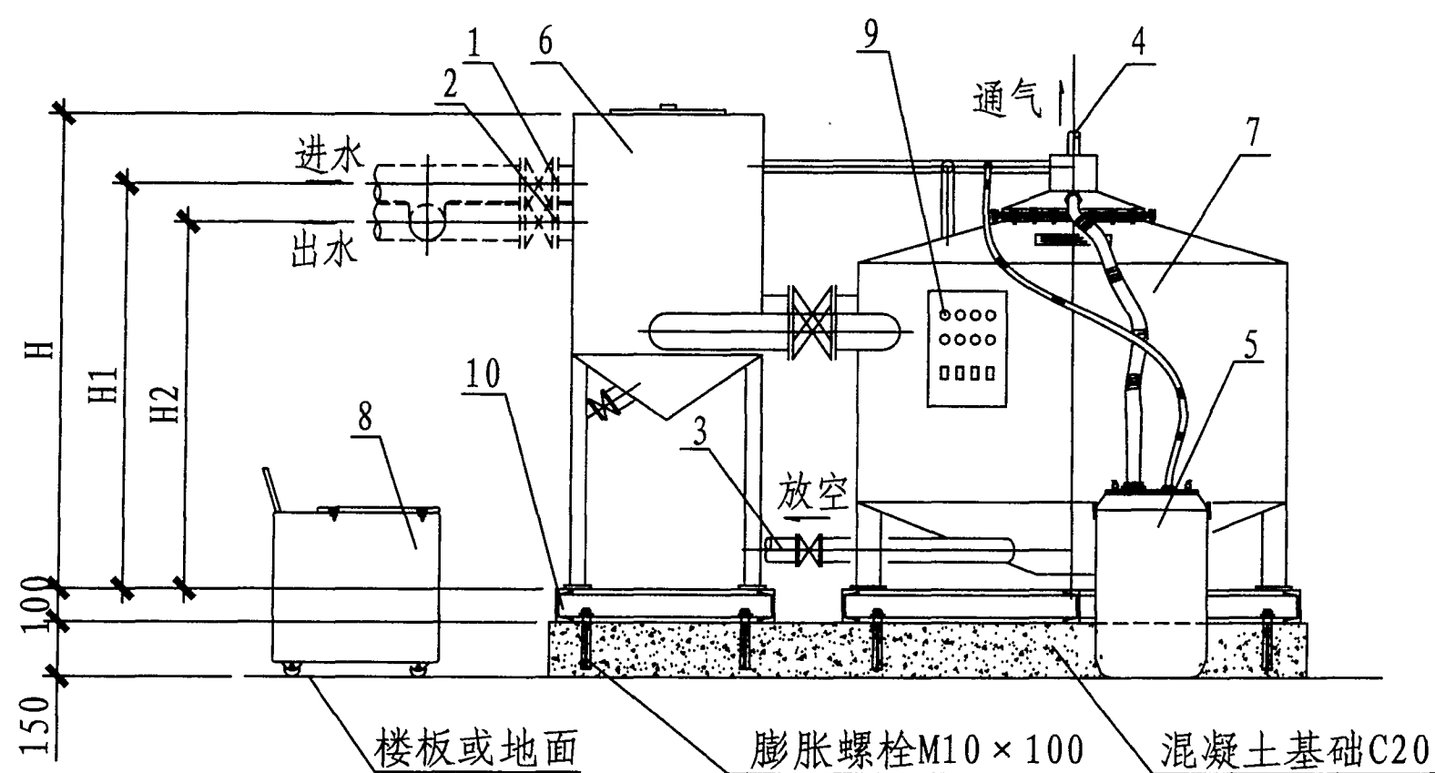
立面图
