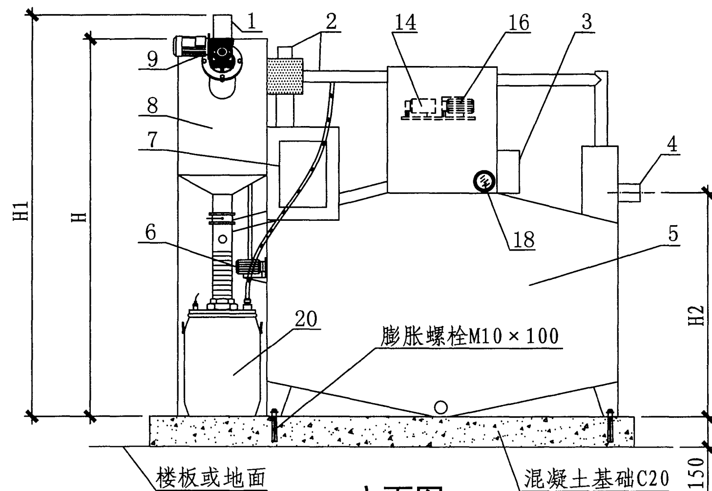
立面图
