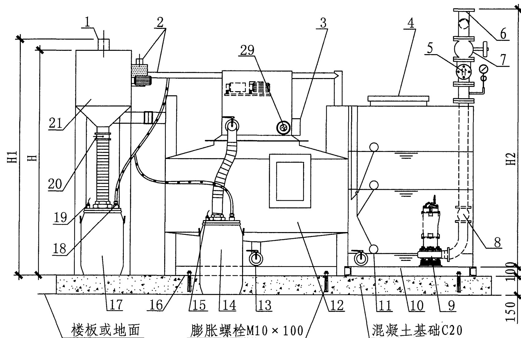
立面图
