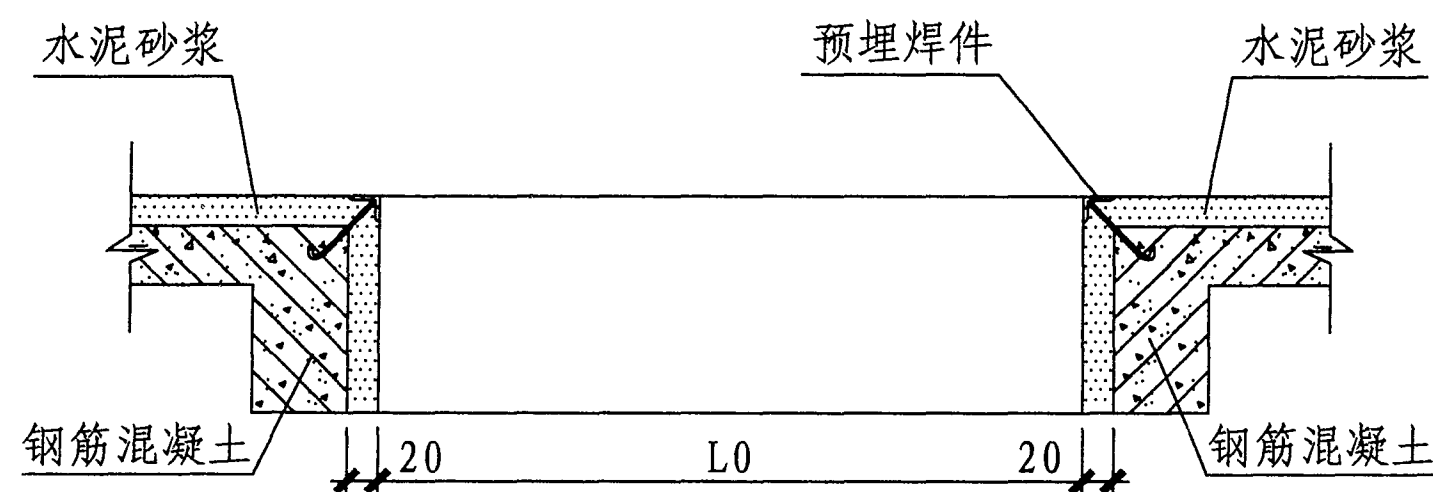
预埋件立面图
