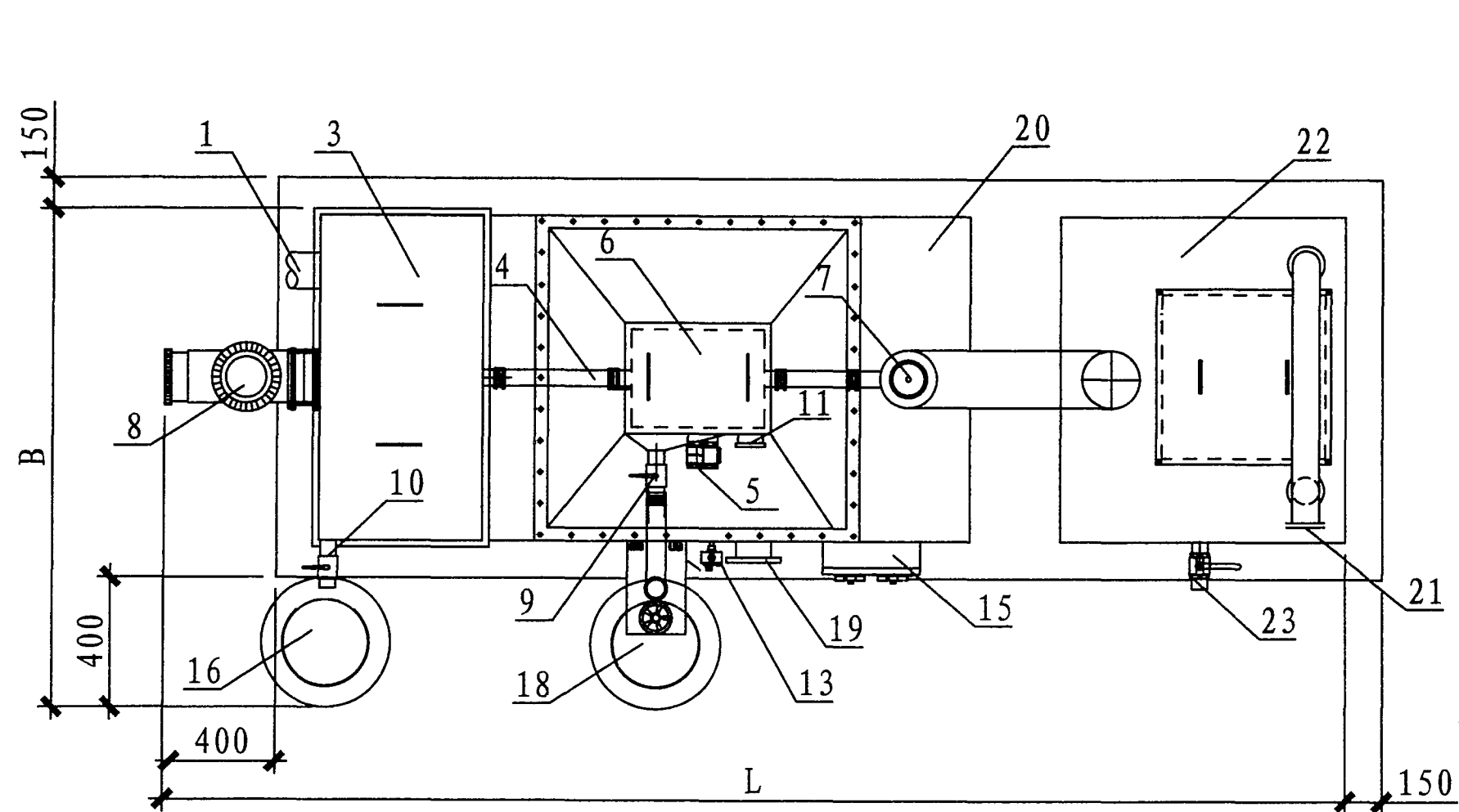
平面图
