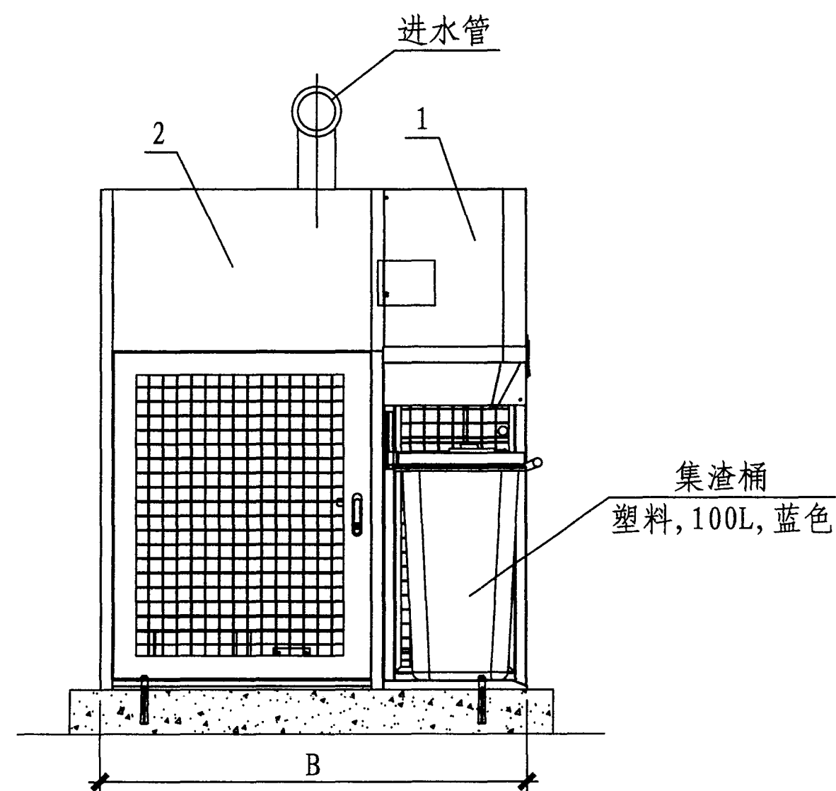
侧面图
