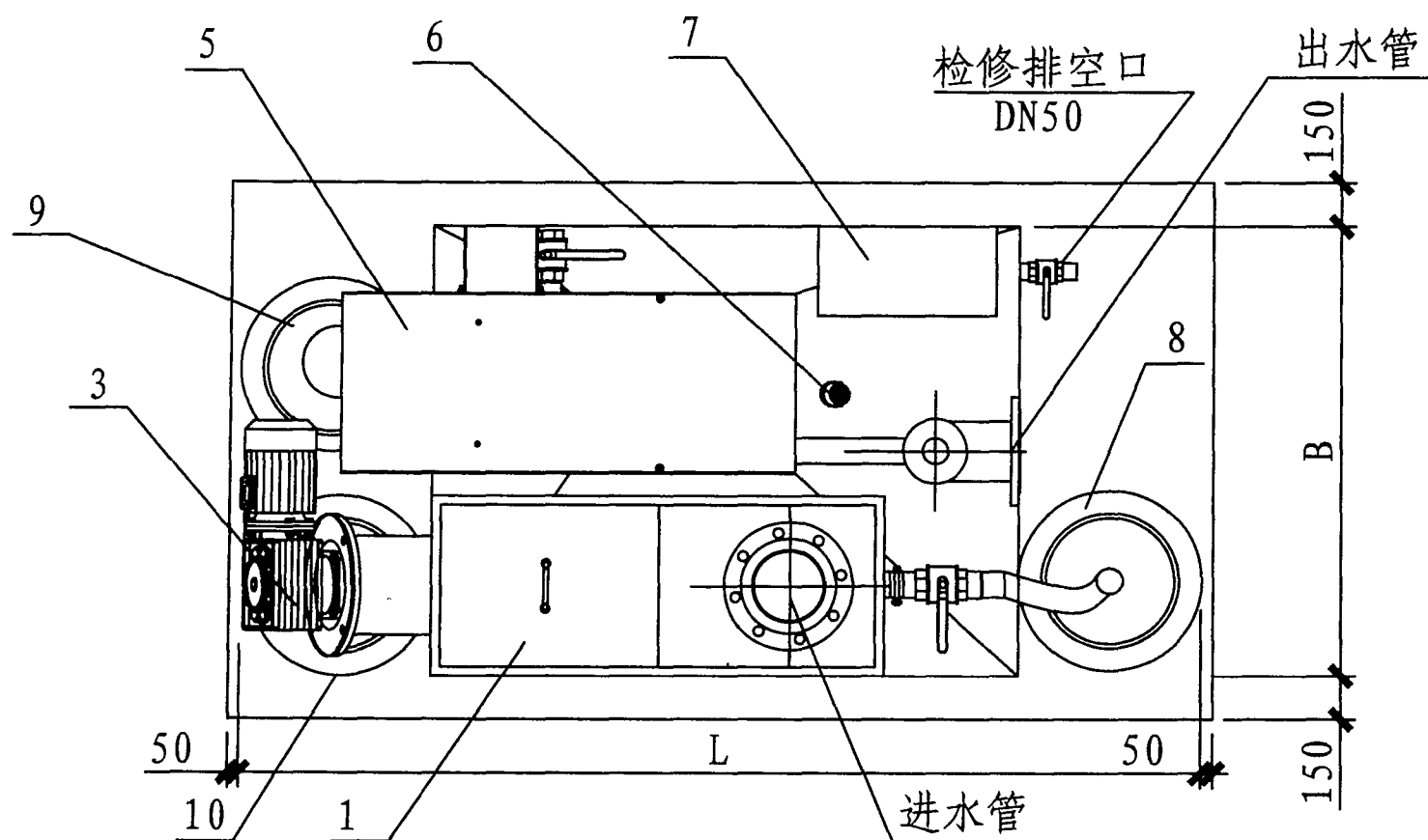
平面图
