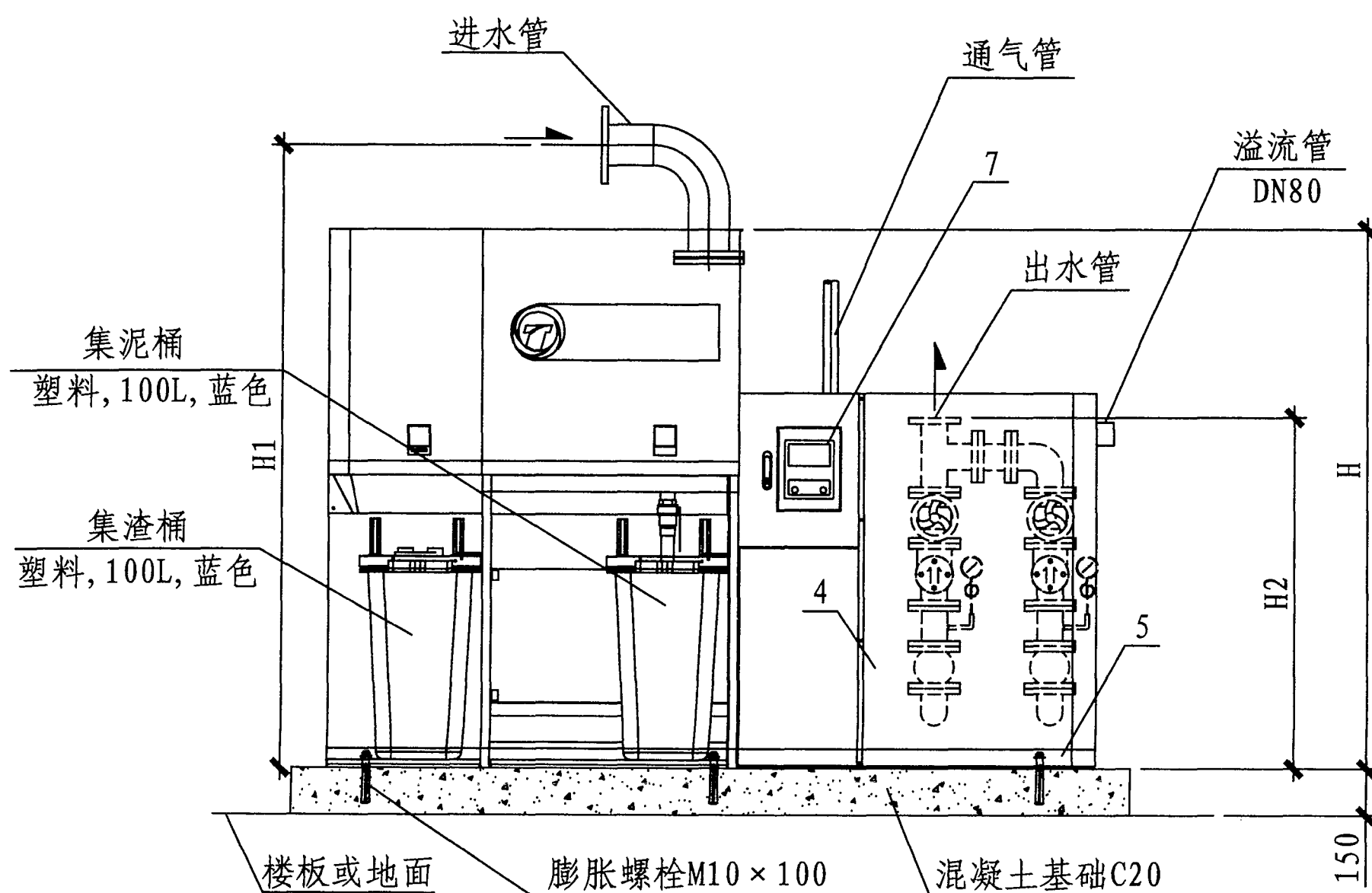
立面图
