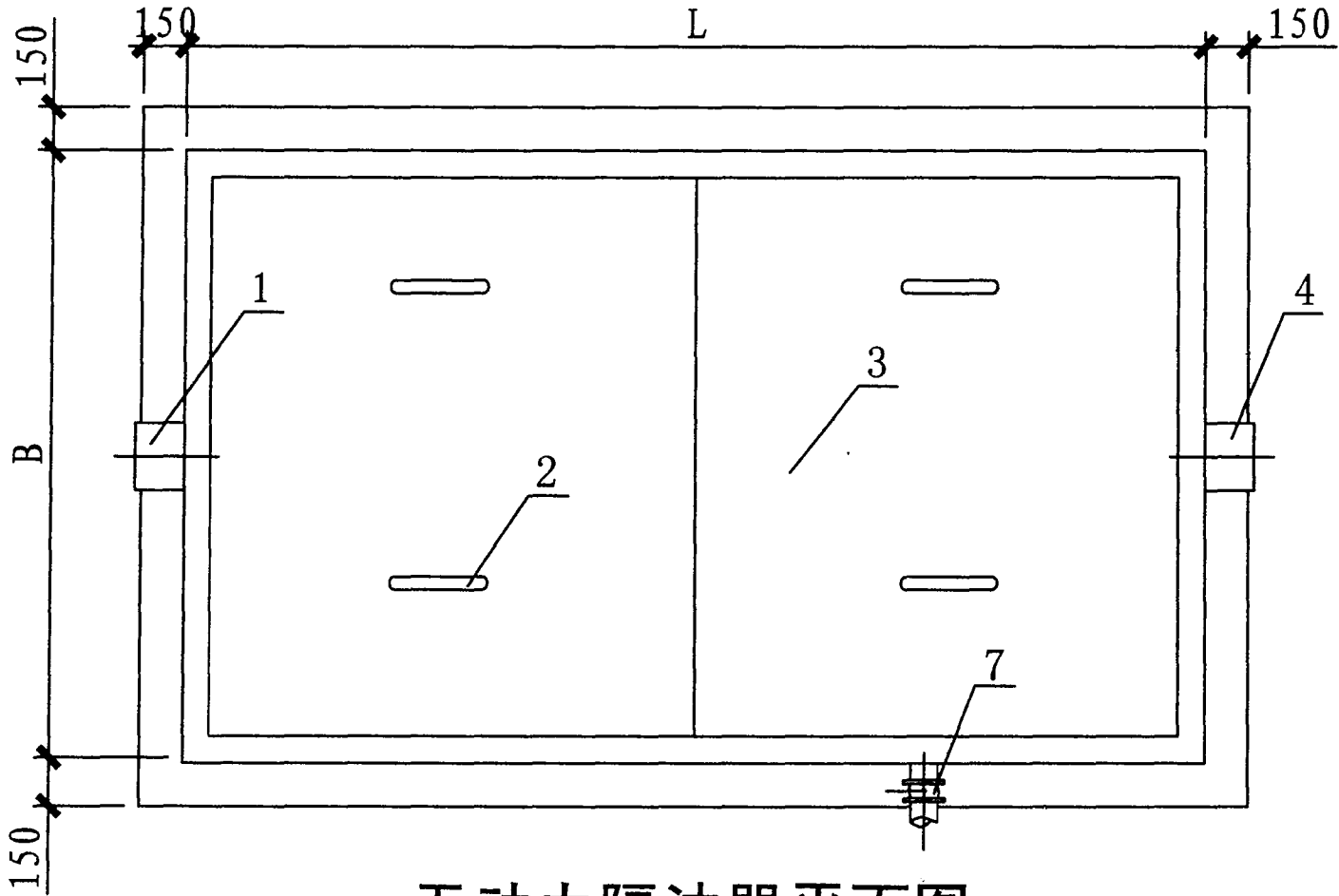
无动力隔油器平面图
