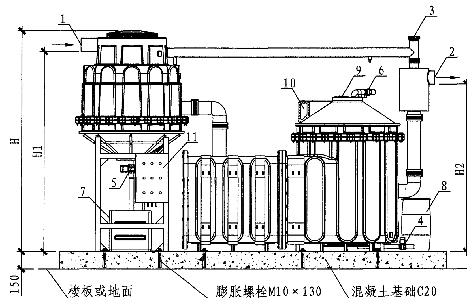
立面图
