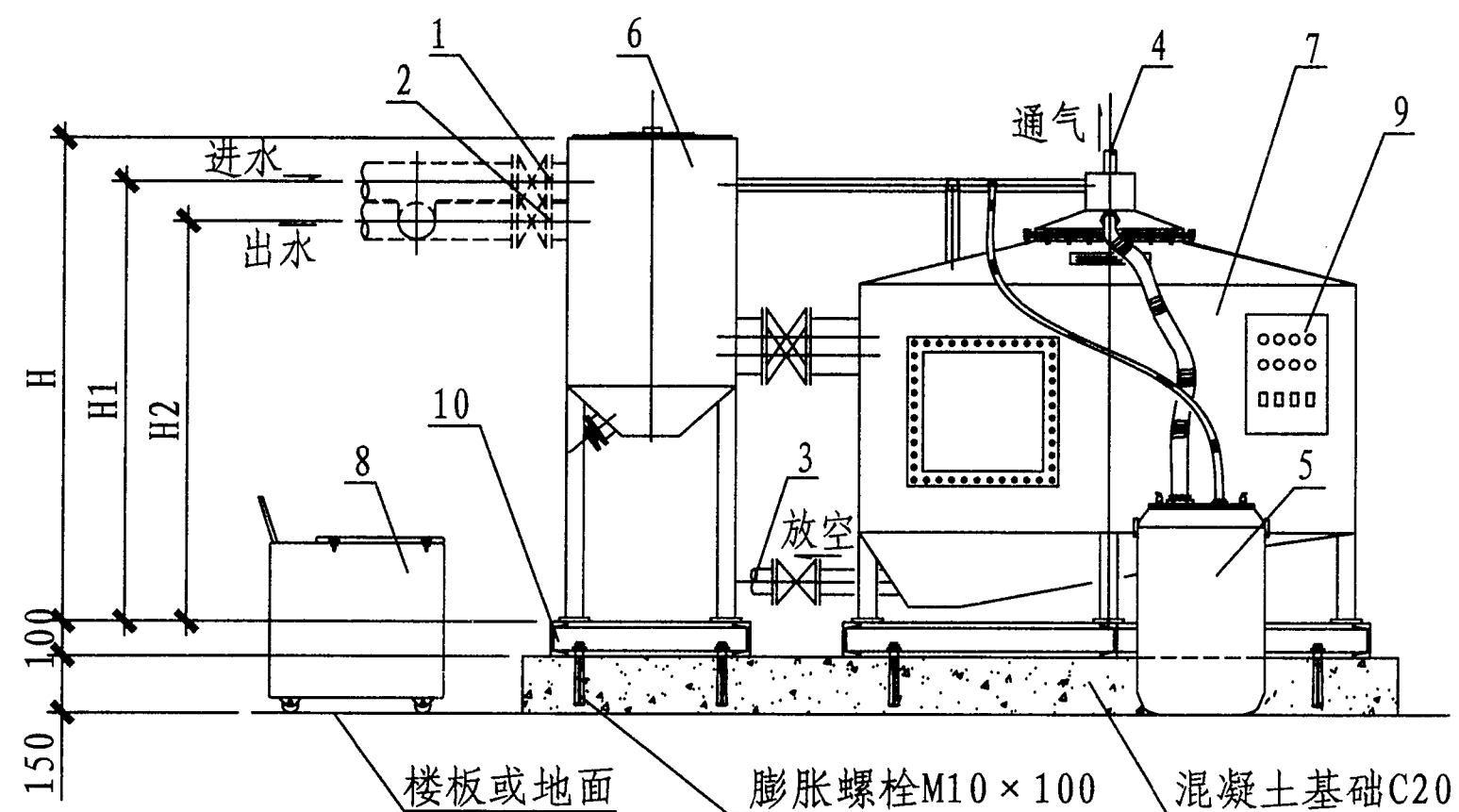
立面图
