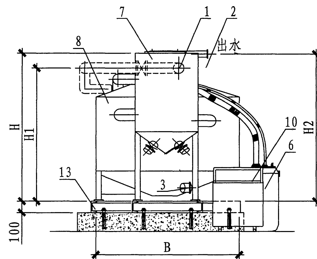
侧面图
