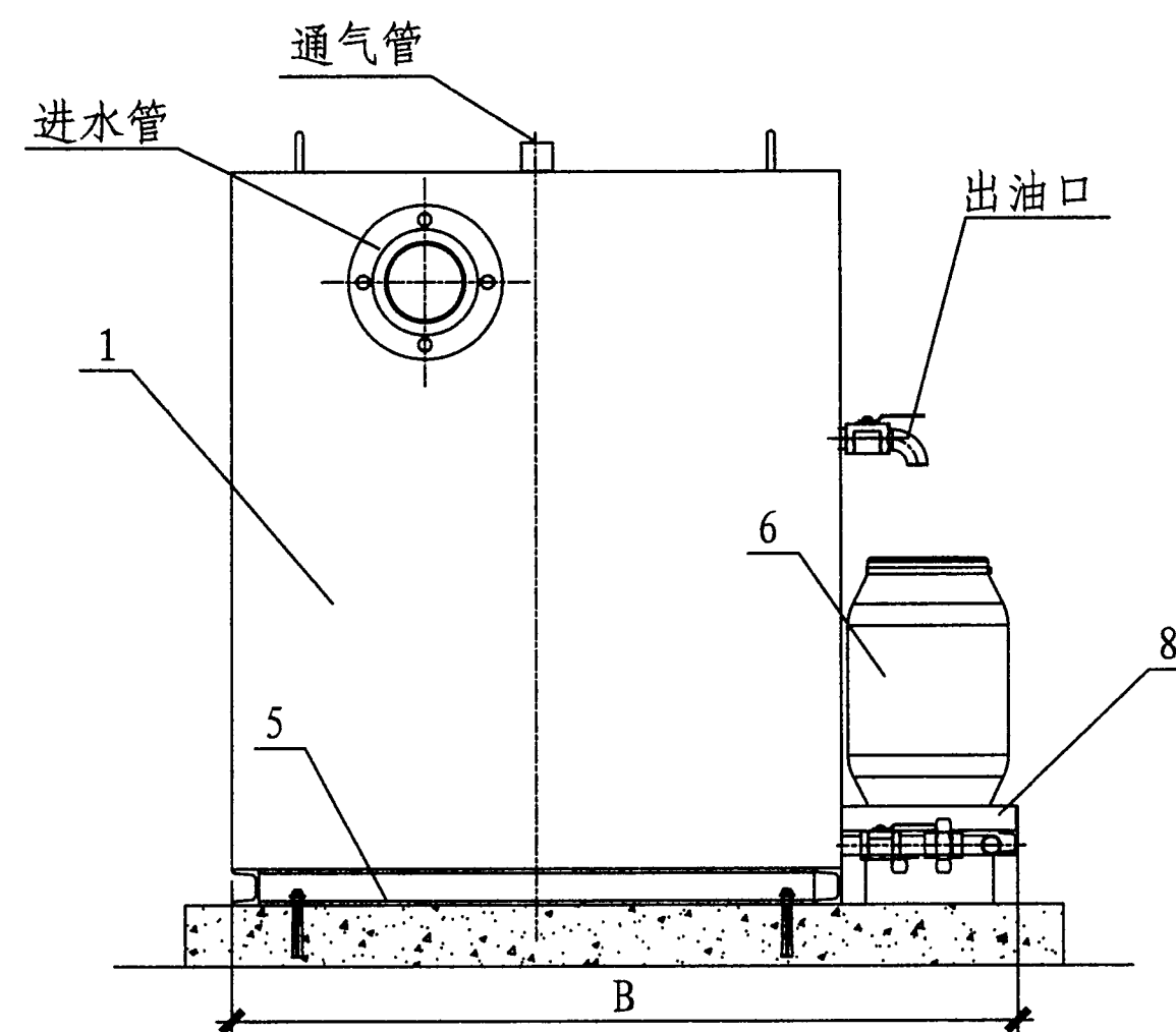
侧面图
