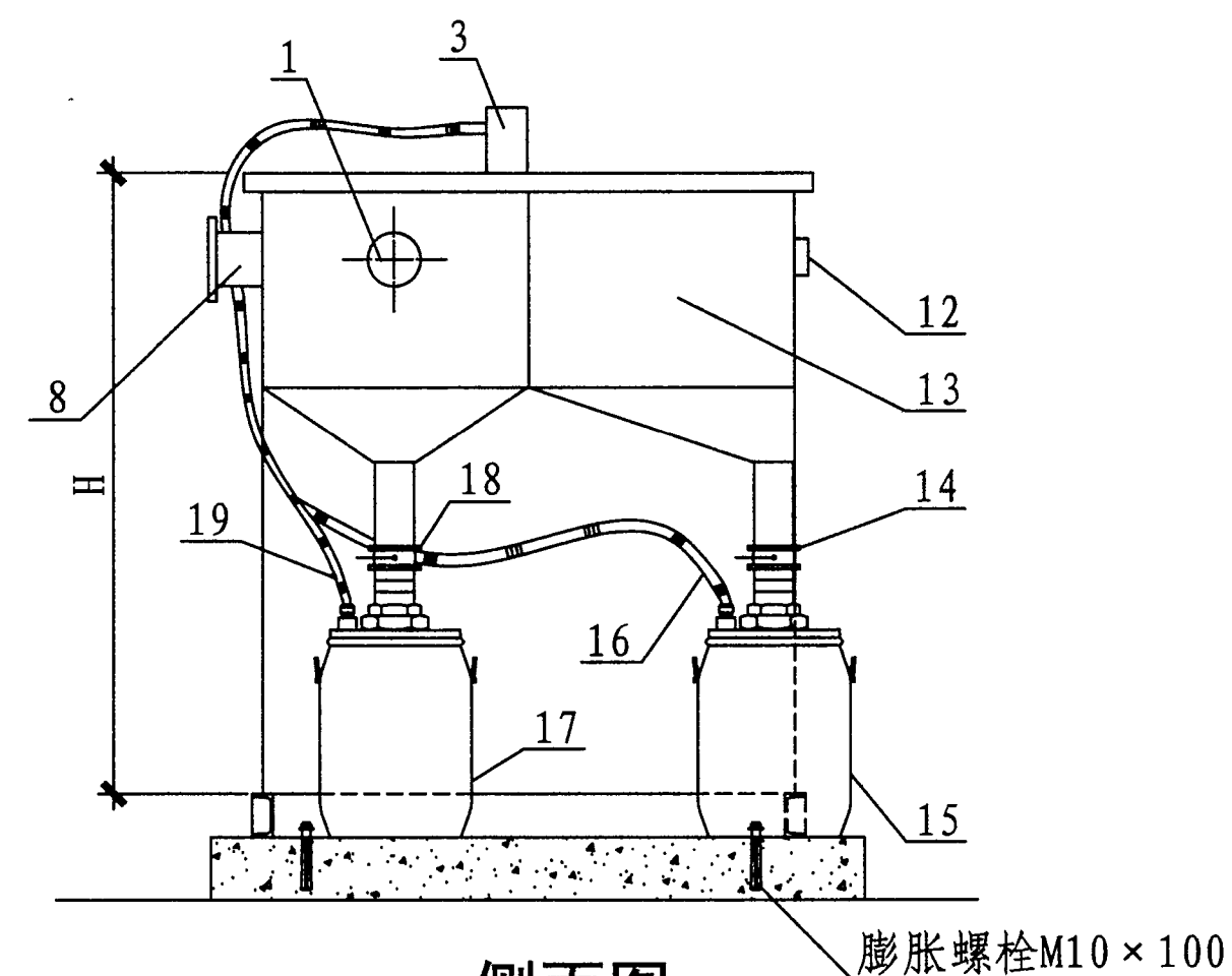
侧面图
