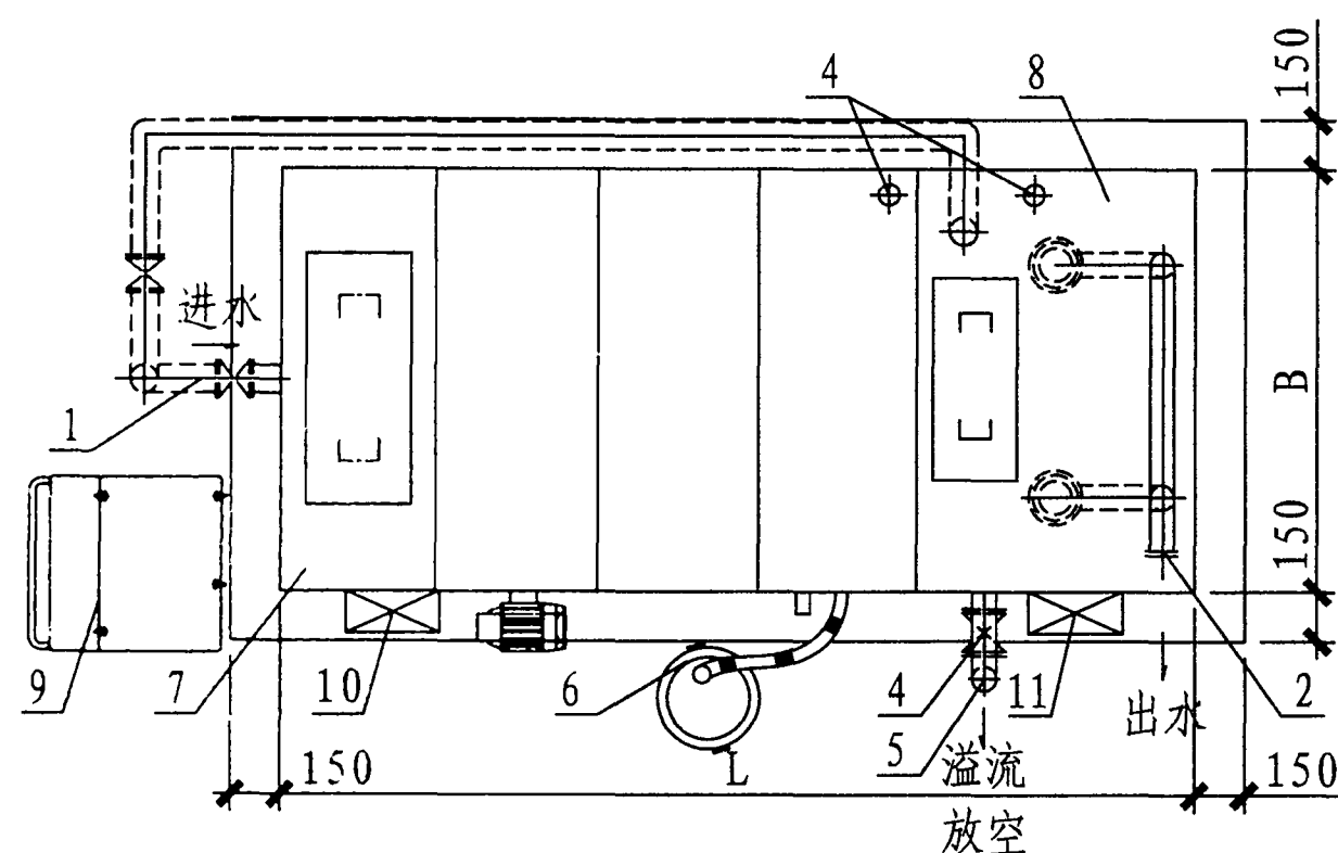
平面图
