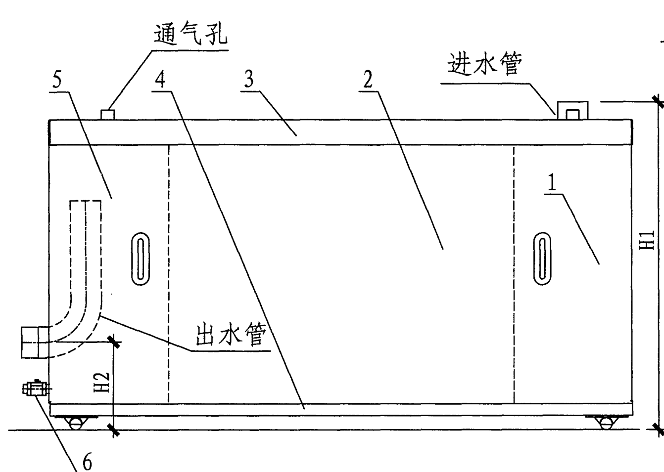
立面图
