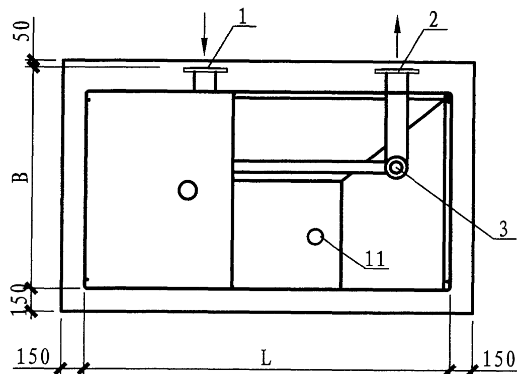
平面图
