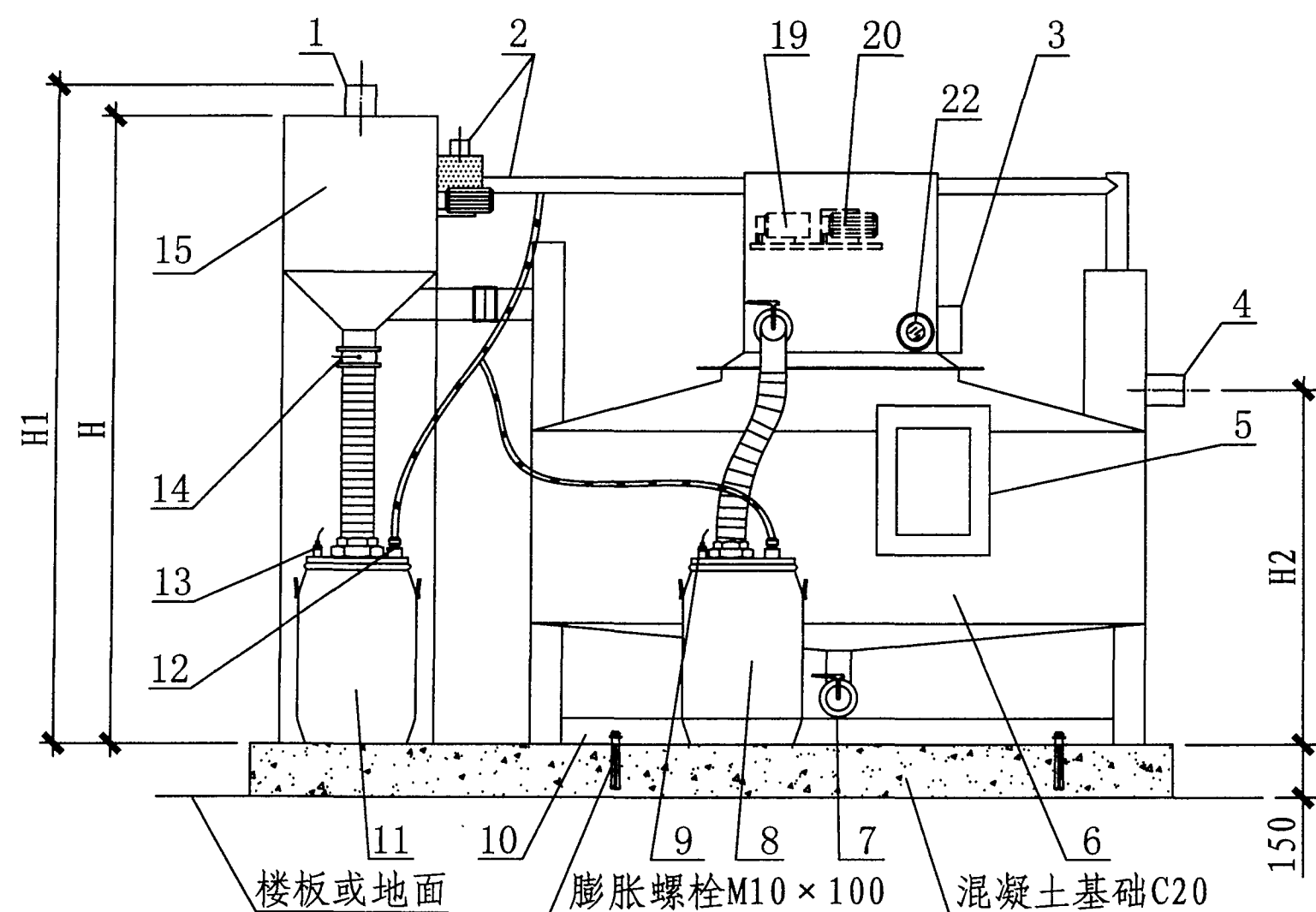
立面图
