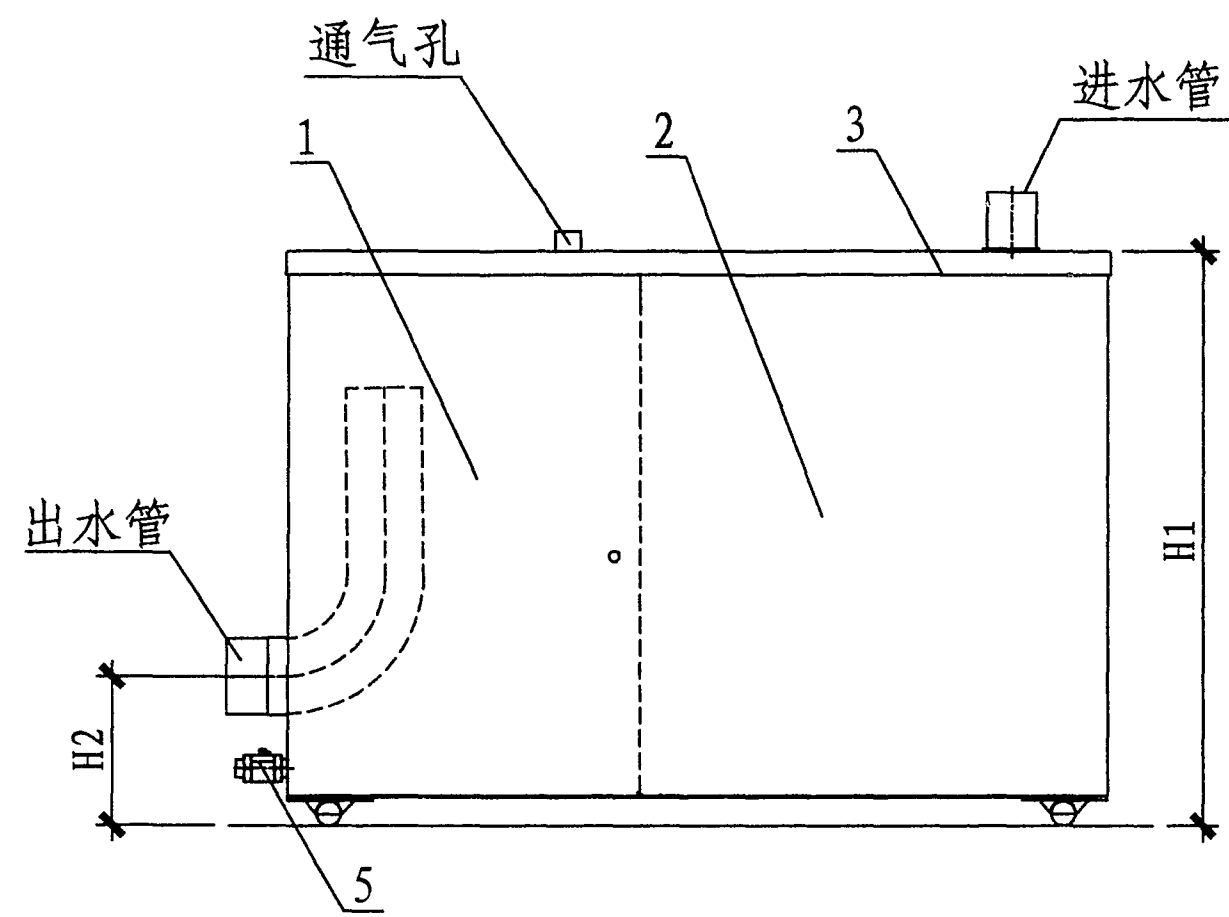
立面图
