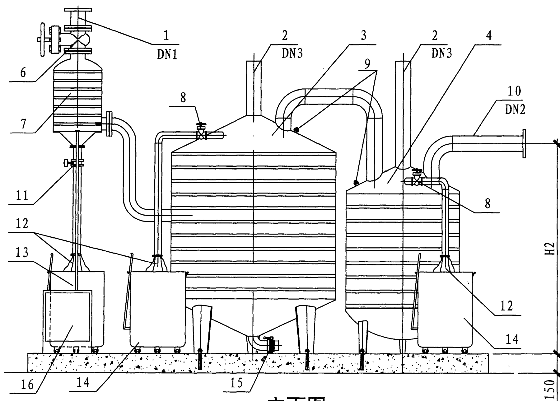
立面图
