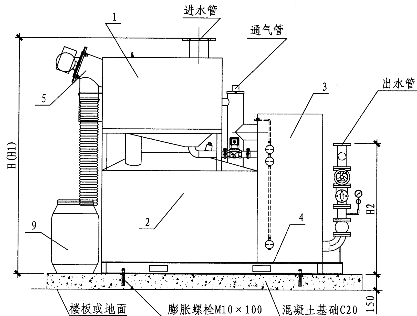
立面图
