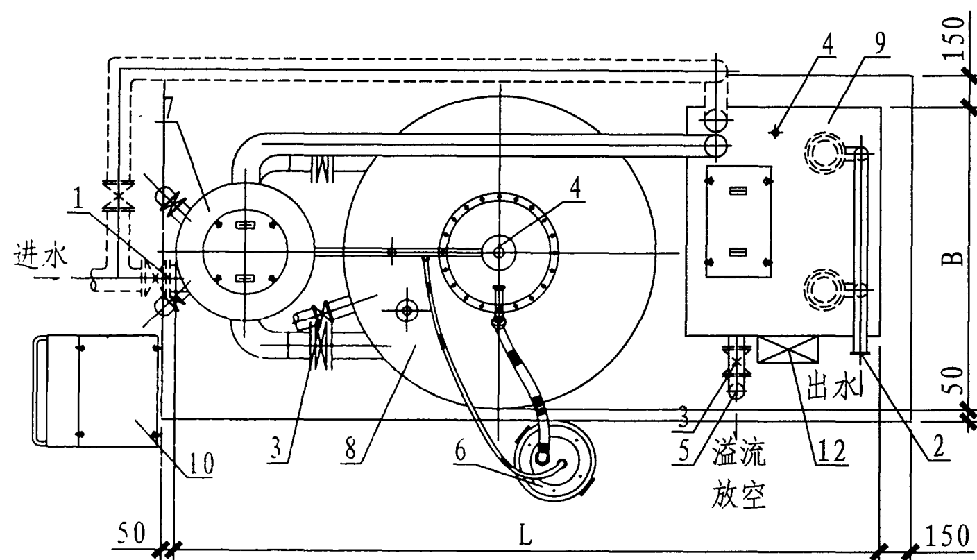
平面图
