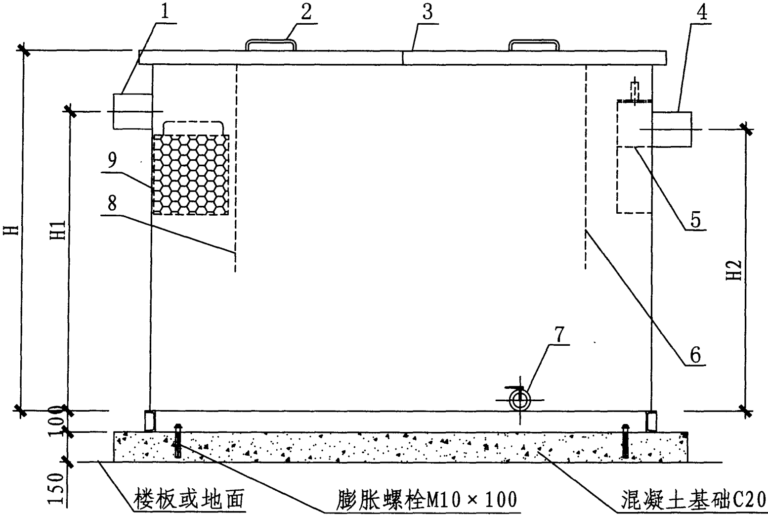
立面图
