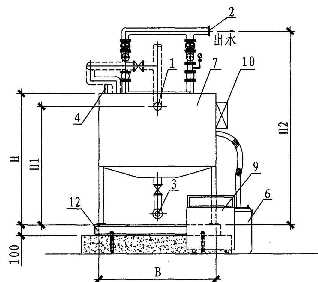
侧面图
