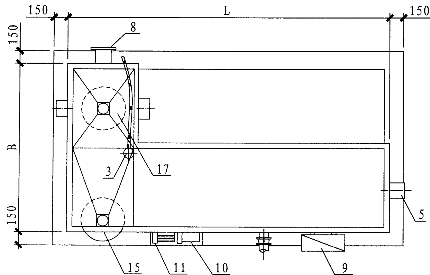
平面图
