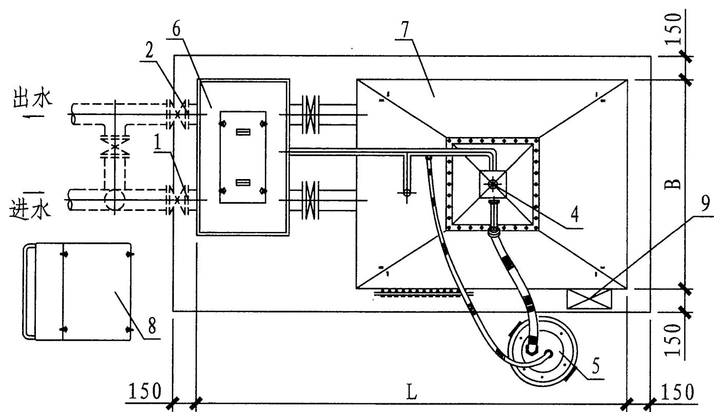
平面图
