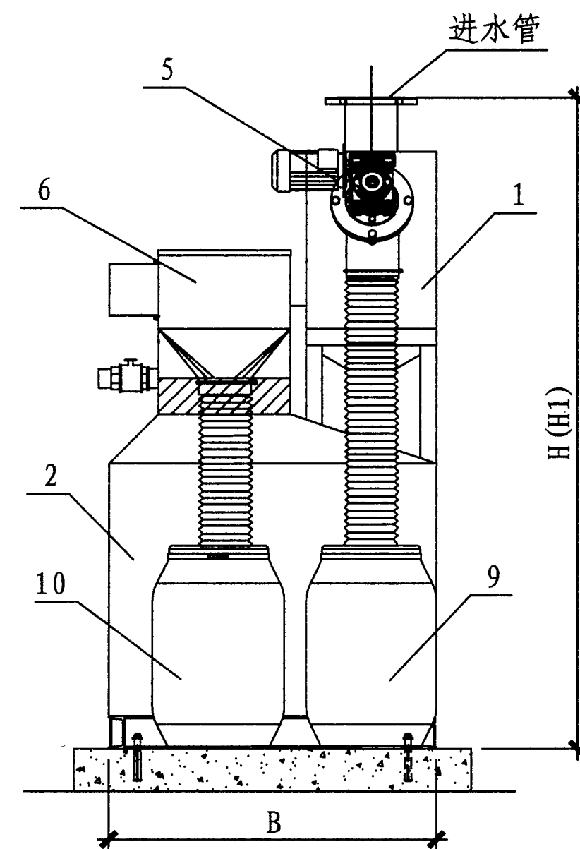
侧面图
