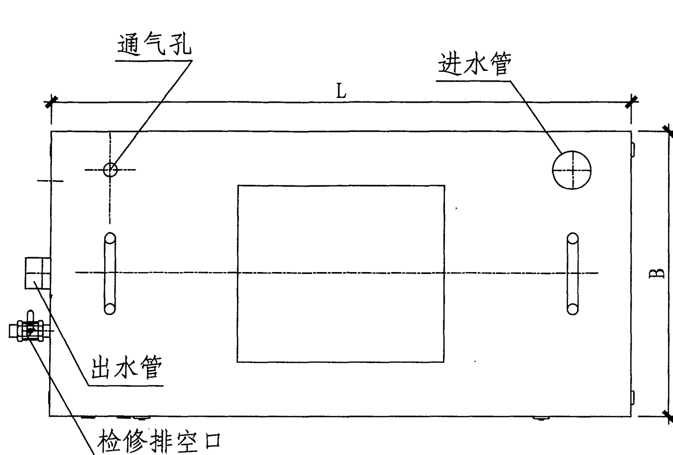
平面图
