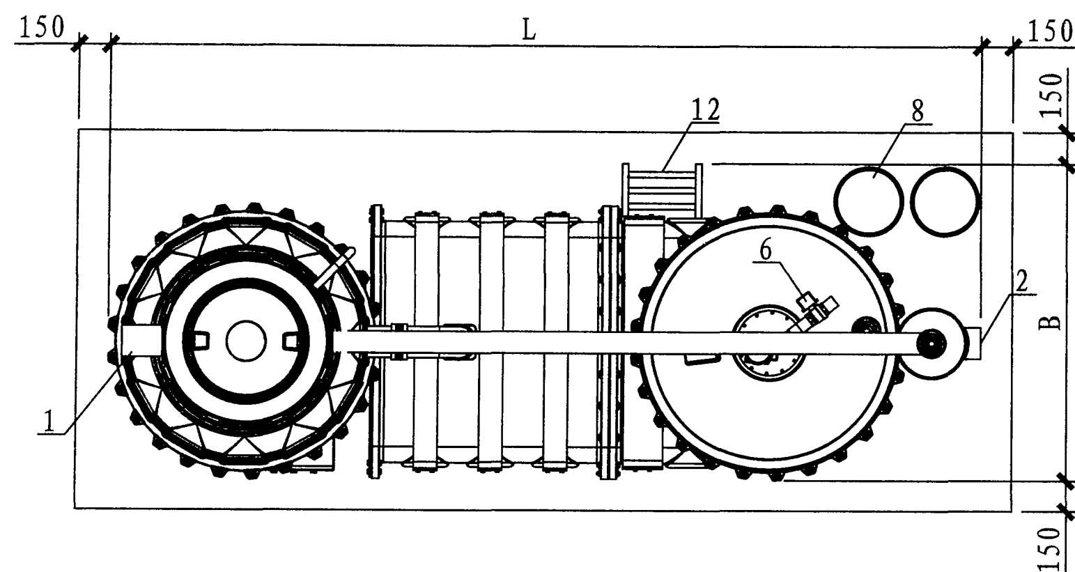
平面图
