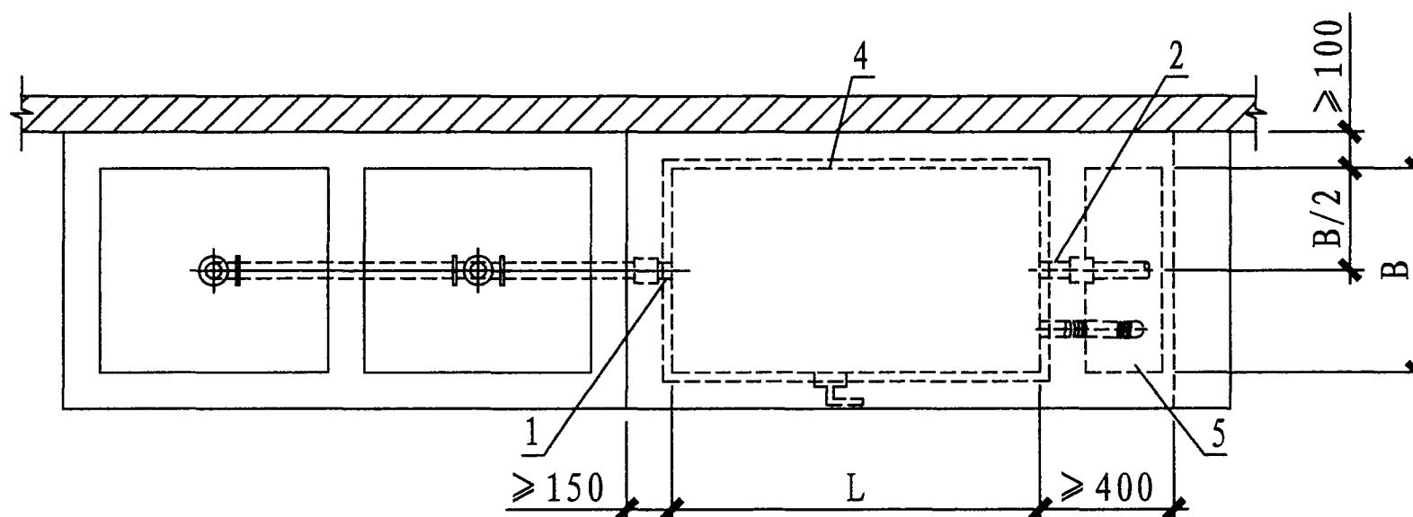
JYGYQ-D2安装平面图
