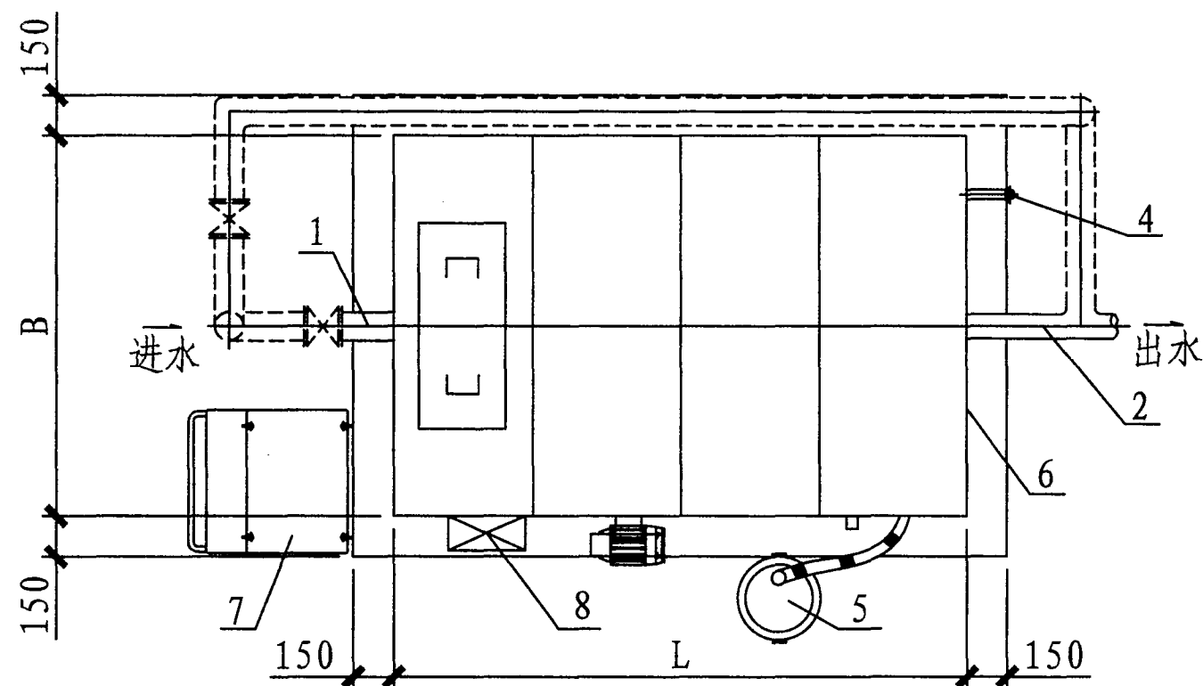
平面图
