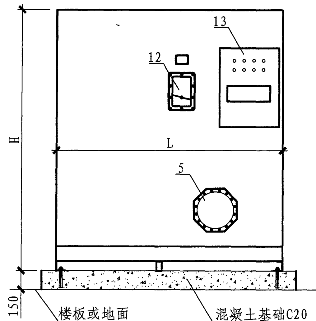
立面图
