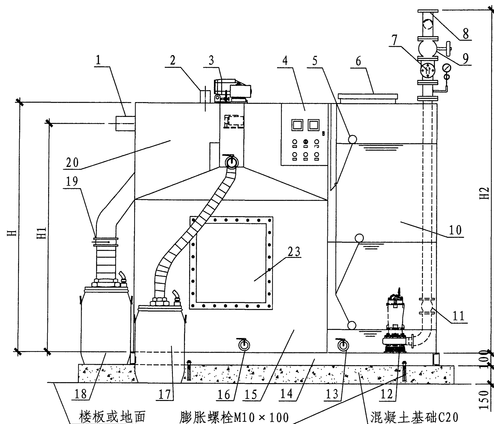
立面图
